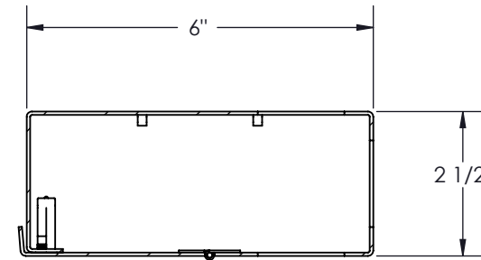
COUPE A-A ÉCHELLE 1 : 3
