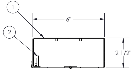
COUPE A-A ÉCHELLE 1 : 4
