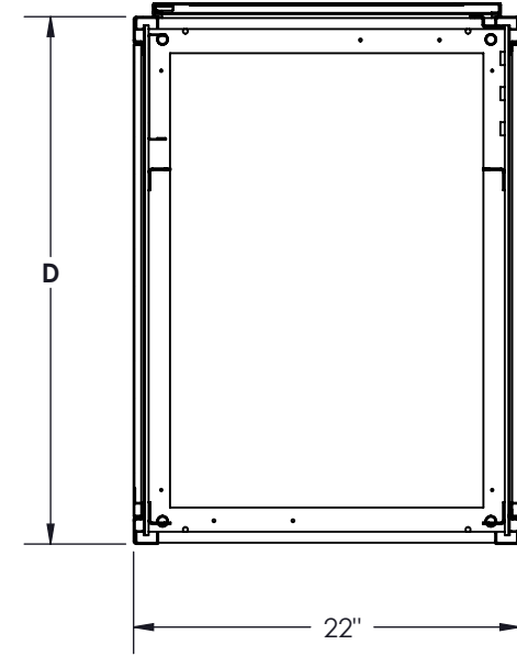
SECTION B-B SCALE 1 : 12
