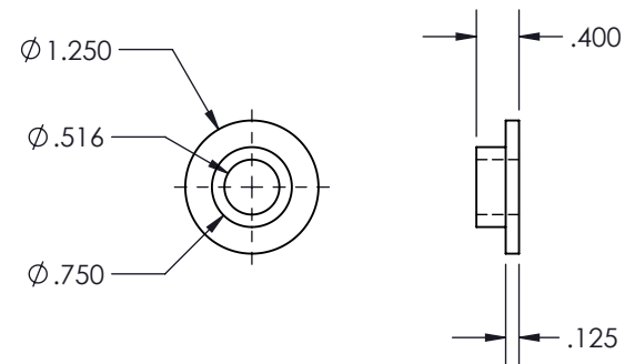
DÉTAIL BAGUE EN NYLON
