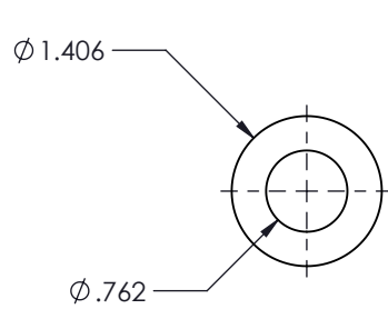
DÉTAIL RONDELLE EN NYLON
