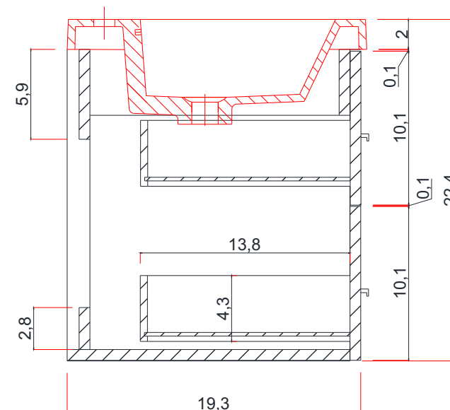
B-B KESİTİ
