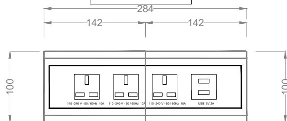
TOP VIEW - DOOR CLOSE
