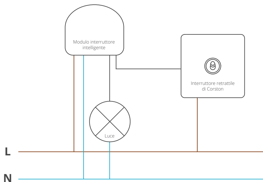
Esempio di cablaggio* (il cablaggio varia tra i moduli)
