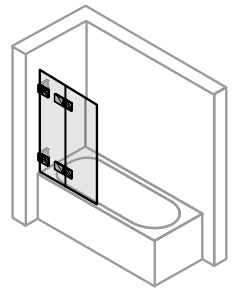
LHC
