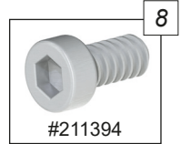
Zylinderschraube DIN 912 M6x14 cylinder head screw DIN 912 M6x14
