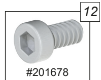
Zylinderschraube DIN 912 M6x12 cylinder head screw DIN 912 M6x12
