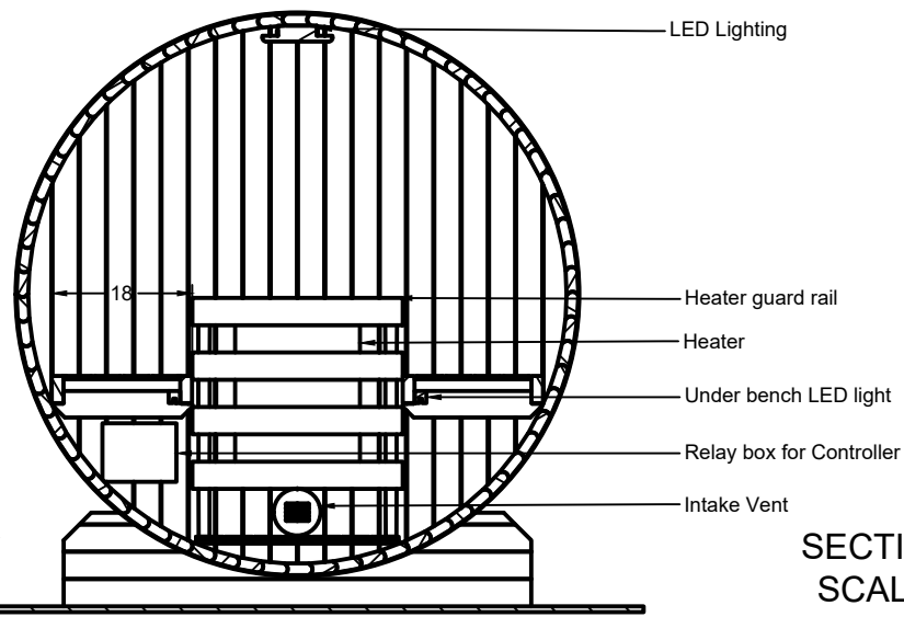
SECTION A-A SCALE 1:27
