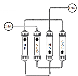
Hybrid UF
