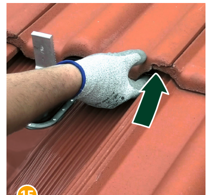
15 Die Blechkantung im Bereich der Ziegel-Überlappung von unten an die Dachpfannen andrücken
