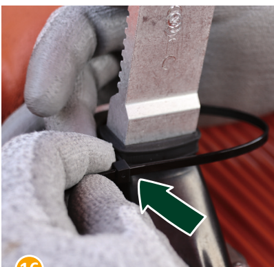
16 Die Oberseite der Dichtmanschette mit Hilfe des Kabelbinders zusätzlich sichern. Die Lasche des Kabelbinders bitte an einer der vier Ecken der Manschette platzieren, festziehen und den überstehenden Rest abschneiden.
