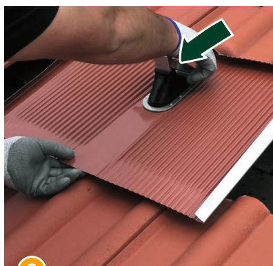
8 Ausparung am Stützblech auf der oberen Querlatte platzieren und Alpha-Platte mit aufgenieteter Dichtmanschette über die Konsolle stülpen
