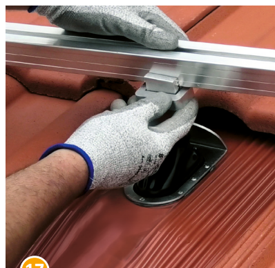
17 Die Klemmkombination wieder auf die Konsole stecken, das Tragprofil auflegen, einhängen, dabei die Höhe durch die Klemmkombination an der Konsole anpassen...
