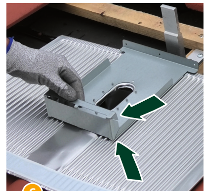
6 Alpha-Platte in ihrer Höhe durch Umfalzen des Stützbleches auf der Rückseite entsprechend anpassen
