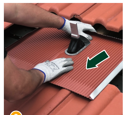
9 Alpha-Platte ausrichten und darauf achten, dass sich im mittleren und oberen Bereich nicht durch unbeabsichtigtes Eindellen Wassersäcke bilden, welche den Wasserabfluß behindern können
