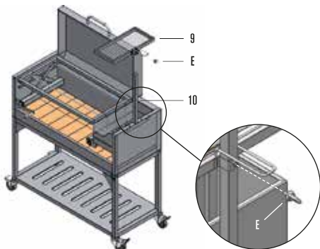
Paso 11 Inserte la parrilla secundaria (9) en el riel lateral ya ensamblado (10) y ajústelo con la tuerca anillada (E).
