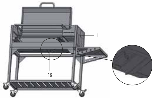
Paso 7 Deslice el sistema de drenaje (16) debajo del cuerpo principal (1).
