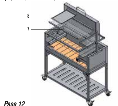
Paso 12 Coloque la parrilla principal (7) y/o la plancha (8) sobre el marco de parrilla principal (1).
