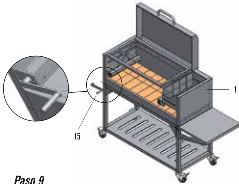
Paso 9 Ensamble la manivela del sistema de ajuste de altura (15) con el cuerpo principal utilizando un tornillo de apriete hexagonal (D).
