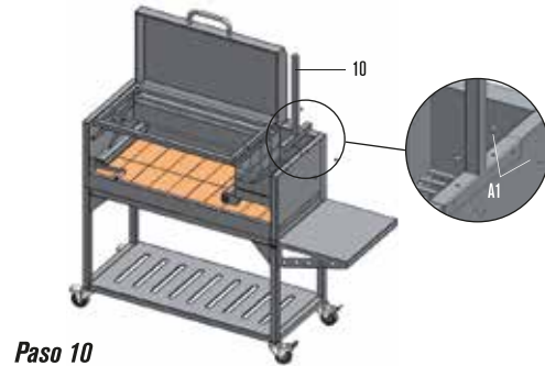
Paso 10 Coloque riel lateral para parrilla secundaria (10) en el lateral derecho del brasero usando cuatro tornillos hexagonales M6*10mm (A1) en la parte inferior y con uno en el medio.
