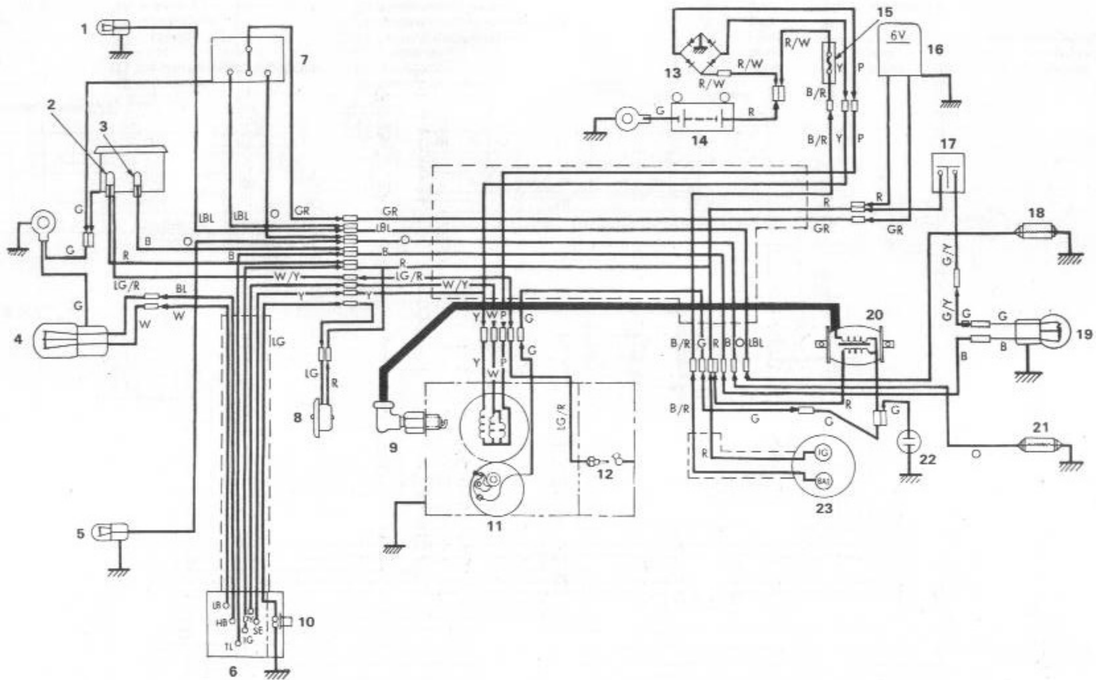
Bild 272 Verdrahtungsschema C90
