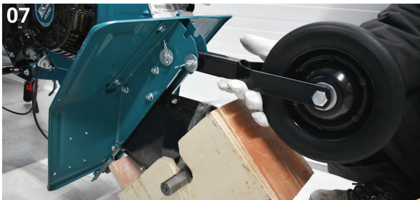
Мал.7. Загальний вигляд закріпленого транспортувального колеса.
