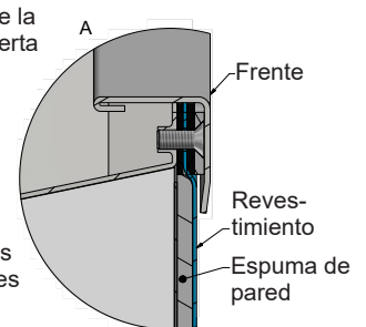
Figura 7. Armazón de bloques aislantes
