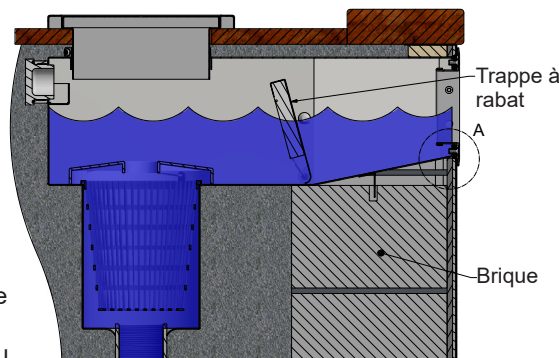
Figure 6. Ossature en brique
