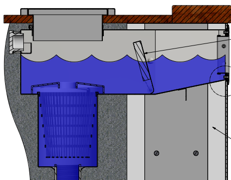
Immagine 7. Vasca in blocchetti isolanti
