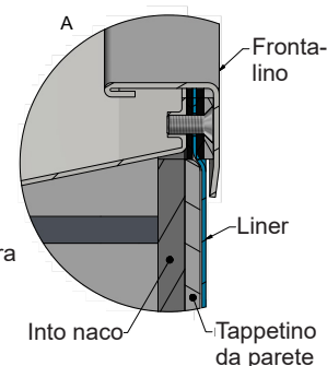
Immagine 7. Vasca in blocchetti isolanti
