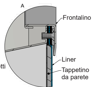
Immagine 7. Vasca in blocchetti isolanti
