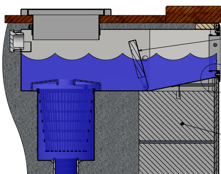
Immagine 6. Vasca in blocchetti Leca
