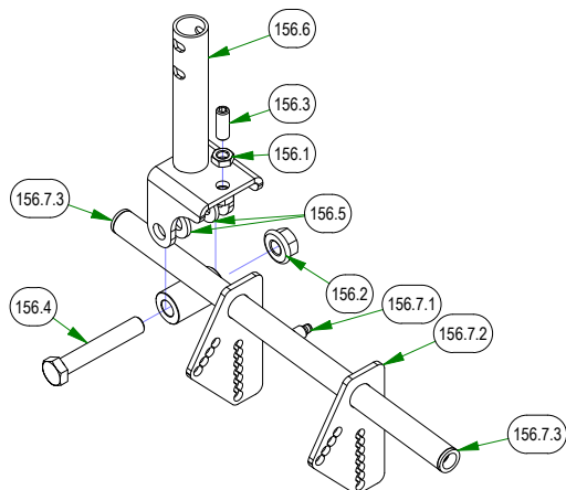
031-0030-19 RH ARM ROD ASSEMBLY
