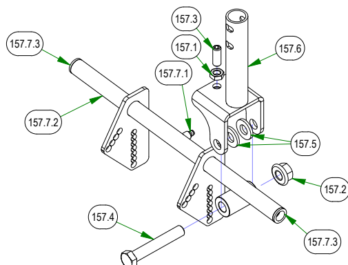
031-0031-19 LH ARM ROD ASSEMBLY
