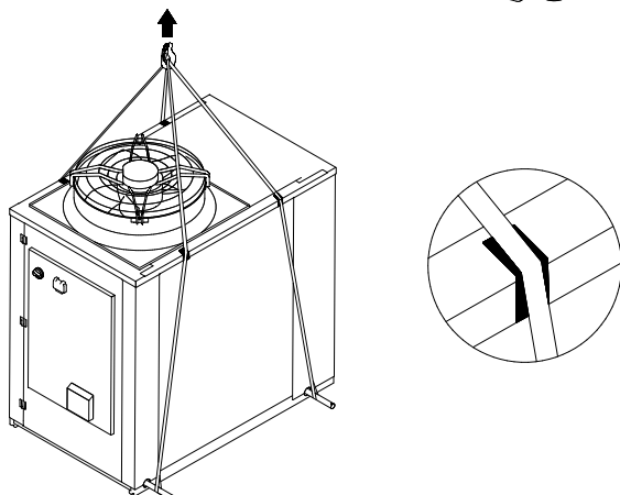
Sollevamento con tubi di sollevamento e funi
