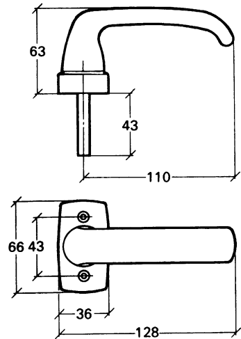
ASSA handtag 17
