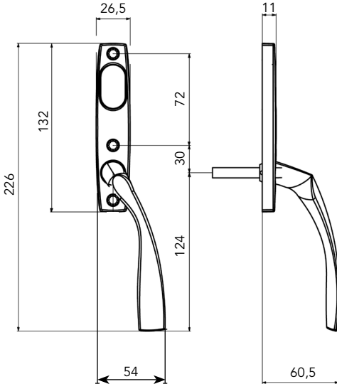
ASSA Vinga 7314/7315
