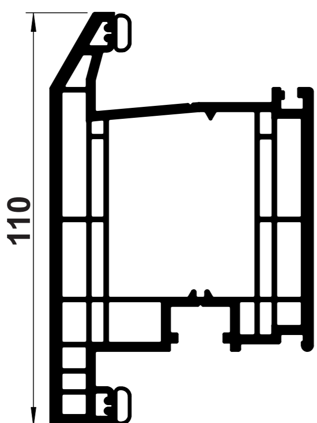
B41 BEVELLED 'T' DOOR SASH
