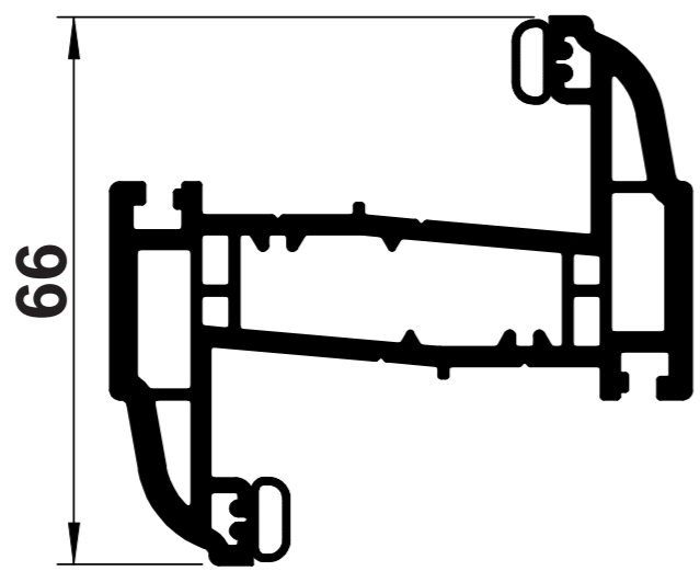
B21 OVOLO SLIM 'Z' TRANSOM
