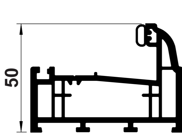
B05 OVOLO SLIM OUTER FRAME
