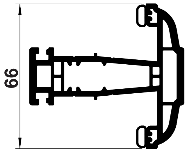
B20 OVOLO SLIM 'T' TRANSOM
