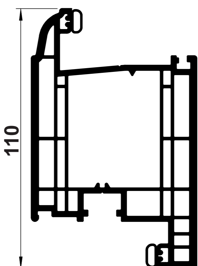
B45 OVOLO 'Z' DOOR SASH
