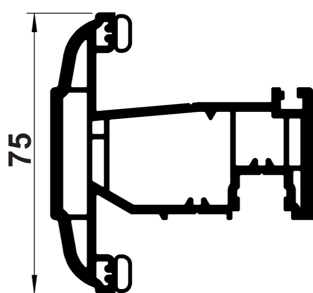
B35 OVOLO 'T' CASEMENT SASH
