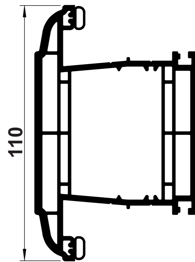
B24 OVOLO 'T' MIDRAIL
