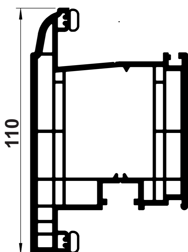
B46 OVOLO 'T' DOOR SASH
