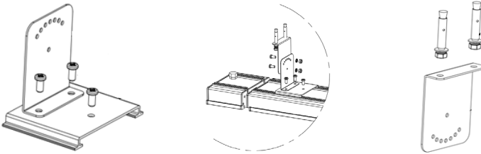
Diagrama 1: Montaje del soporte giratorio
