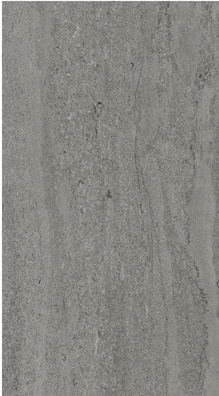
Pumice
