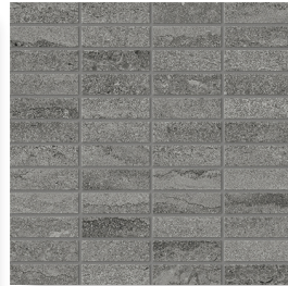
Pumice
