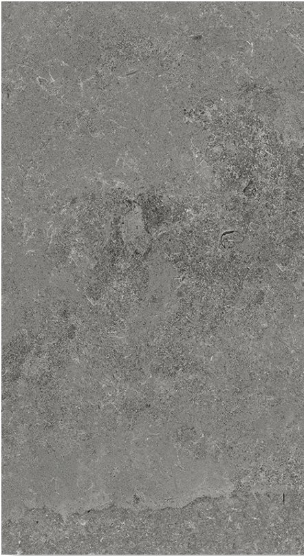
Pumice
