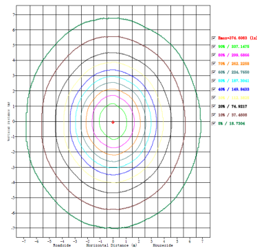
90° (Standard)
