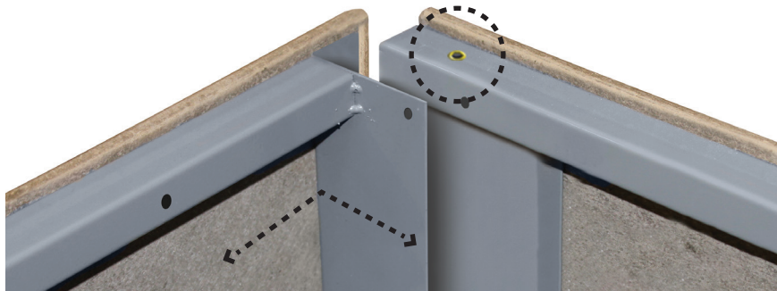
Fig. 13 90° Flange + Nutsert
