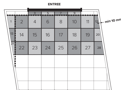
Fig. 3 Sens de pose des dalles INVISIBLE, BUSINESS
