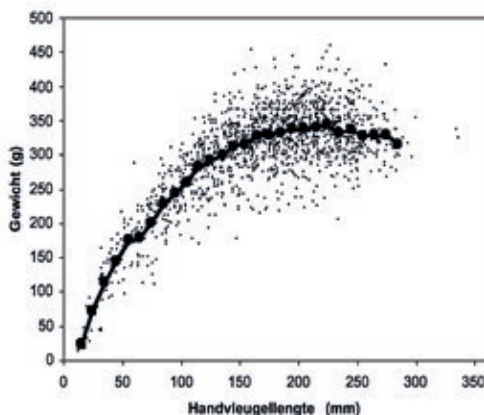
Spreidingscurve gewicht.
