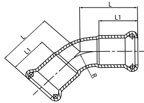
45° ELBOW
