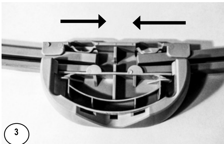
Rail inférieur en résine
