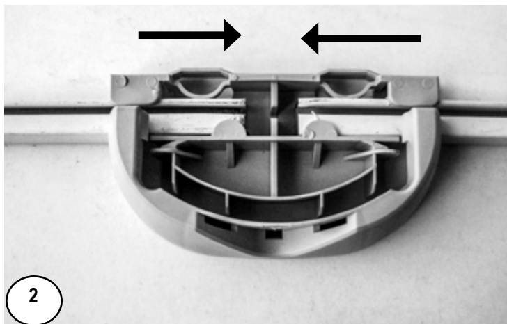
Rail inférieur en acier
