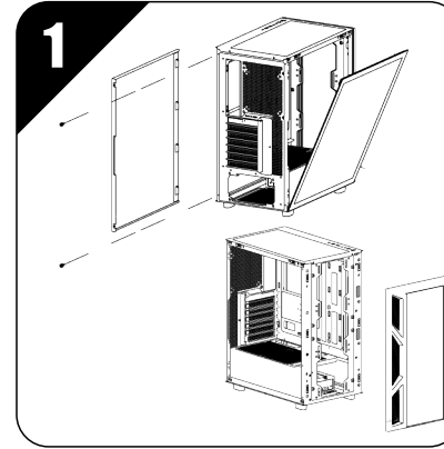
افتح الزجاج الأسير والصفيحة الحديدية اليمنى قم بإزالة اللوحة الأمامية
