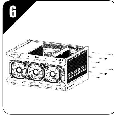
تركيب المروحة السفلية
