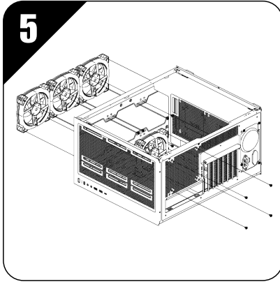
تركيب المروحة الأمامية
