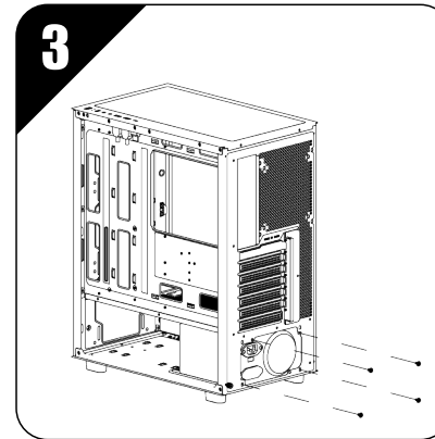
تركيب مصدر الطاقة
