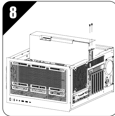
تركيب بطاقة الرسومات
