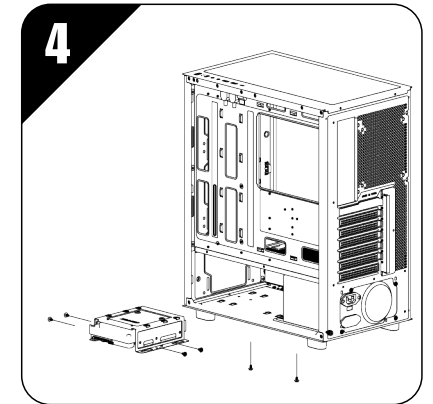
تنصيب محركات الأقراص الصلبة HDD و SSD
