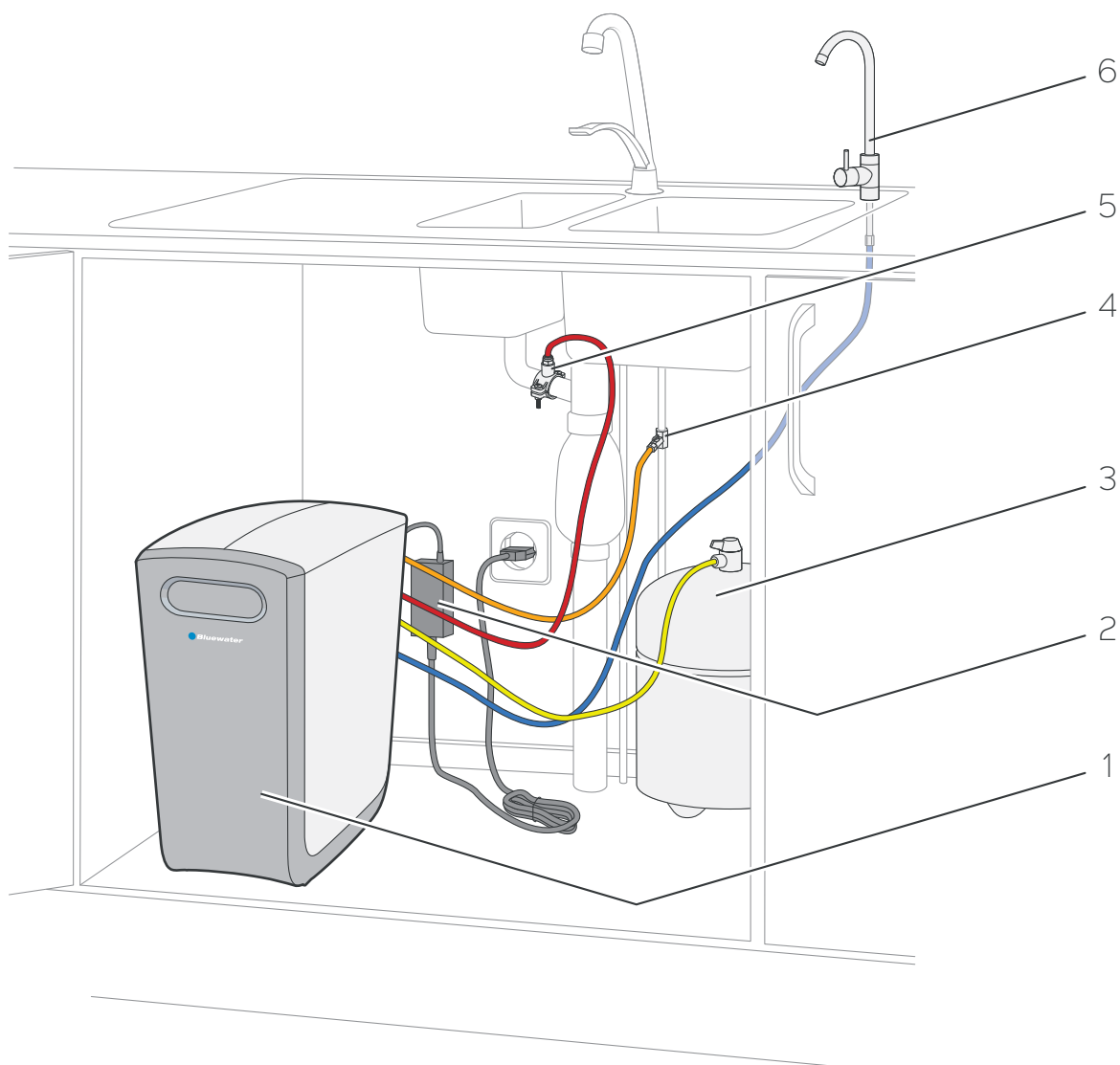
Abbildung 5. Systemübersicht
