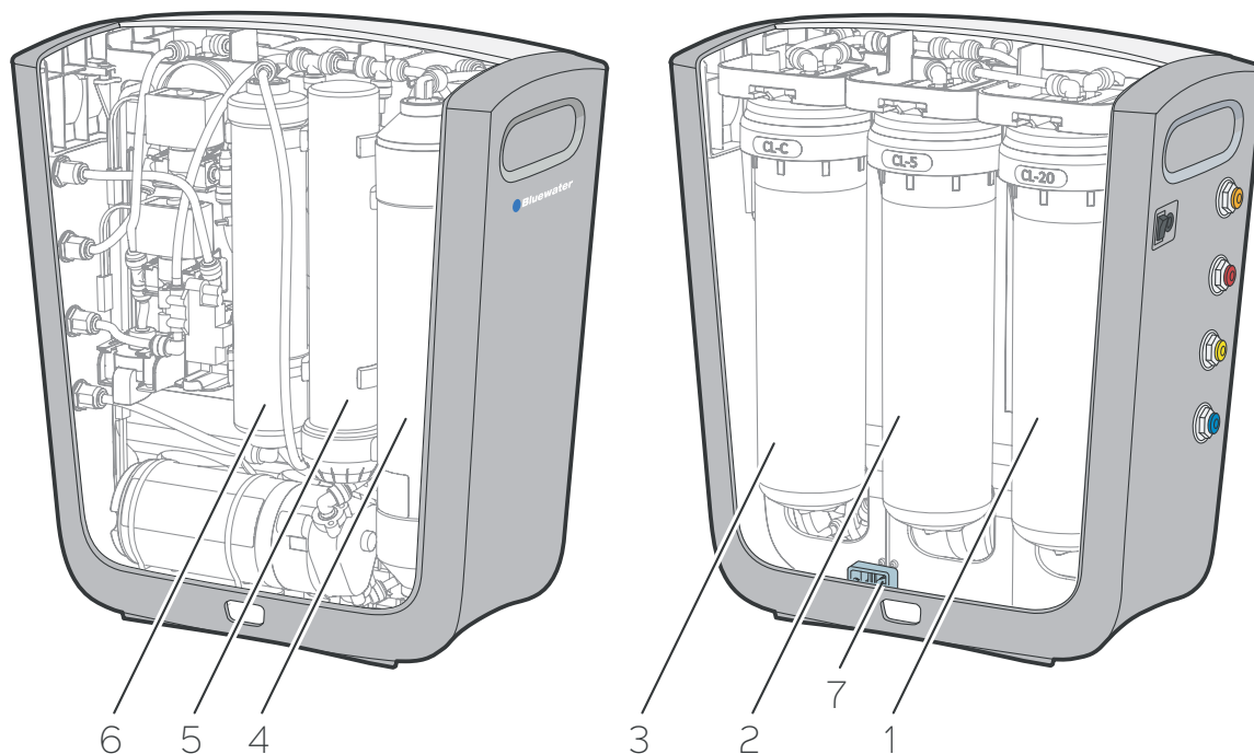
Kuva 4. Cleone sisäpuolelta
