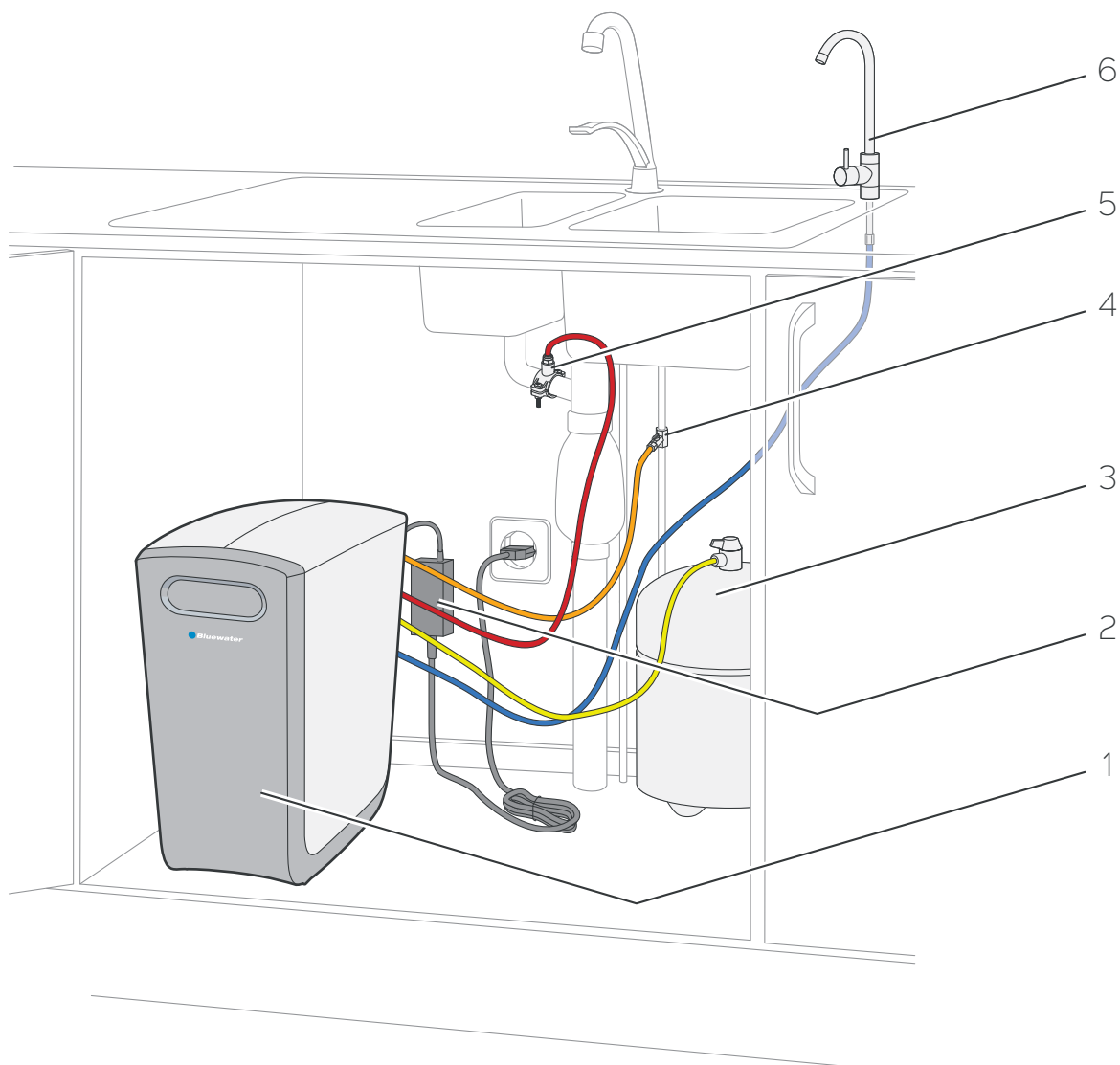
Рисунок 5. Обзор системы
