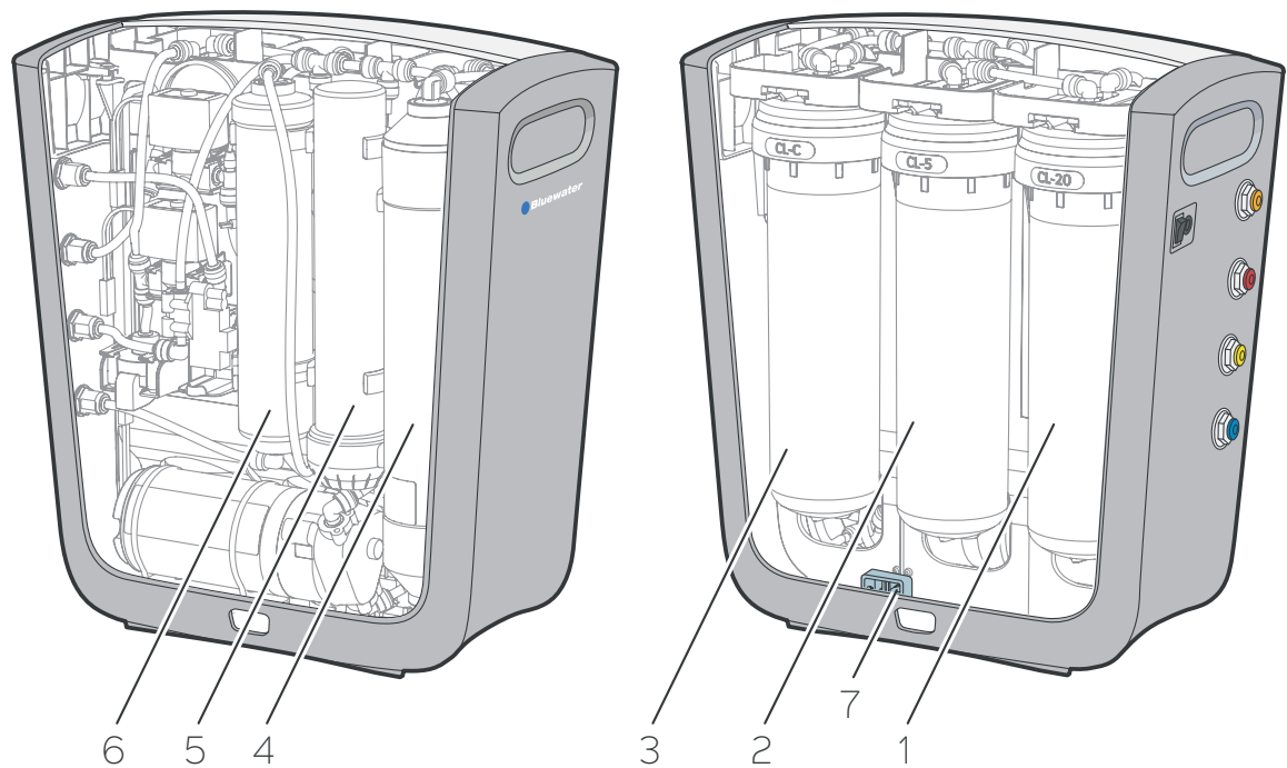
Gambar 4. Cleone dalam
