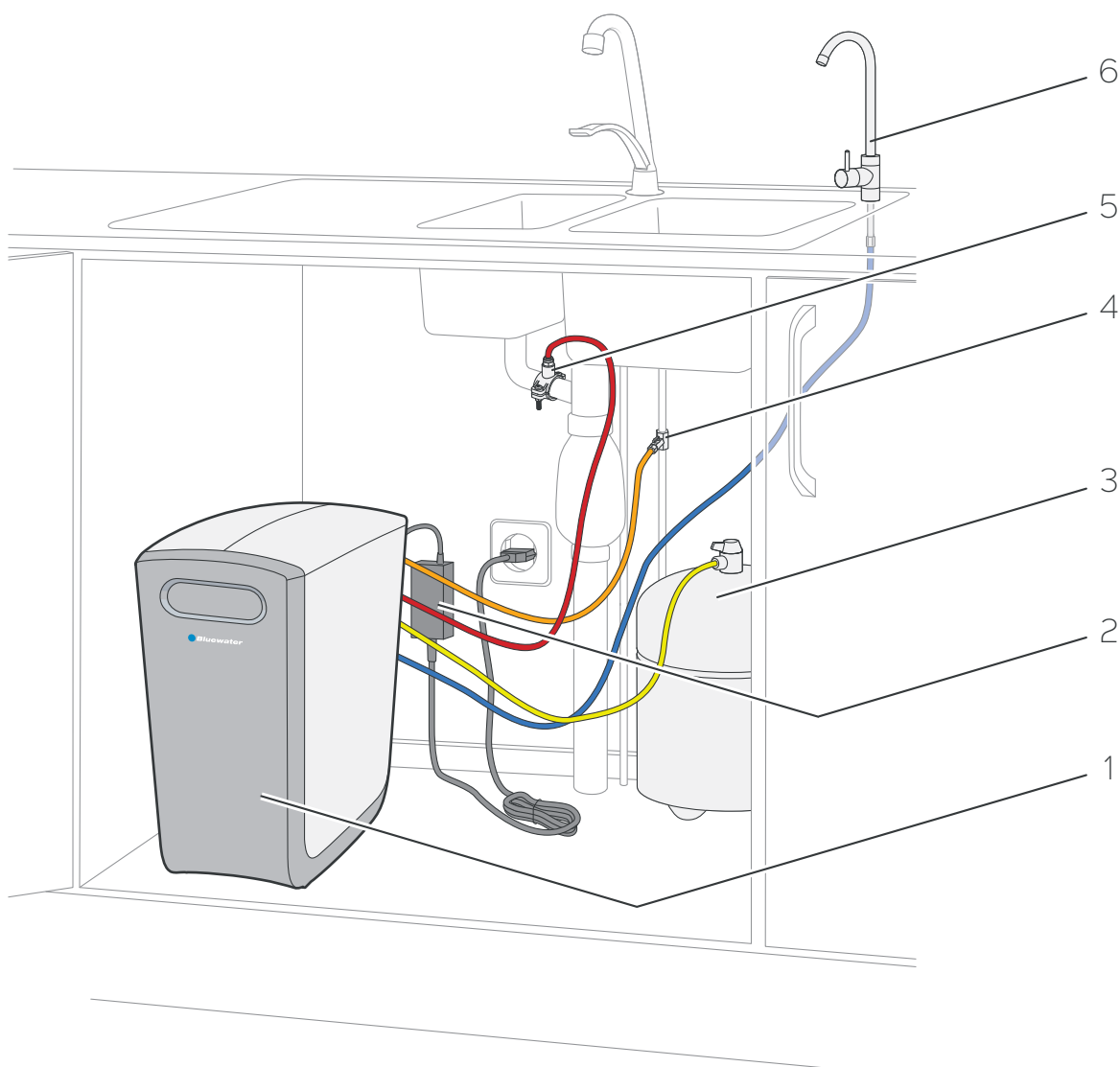
Figur 5. Systemoversikt
