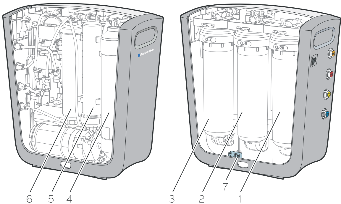
图 4. Cleone 内部
