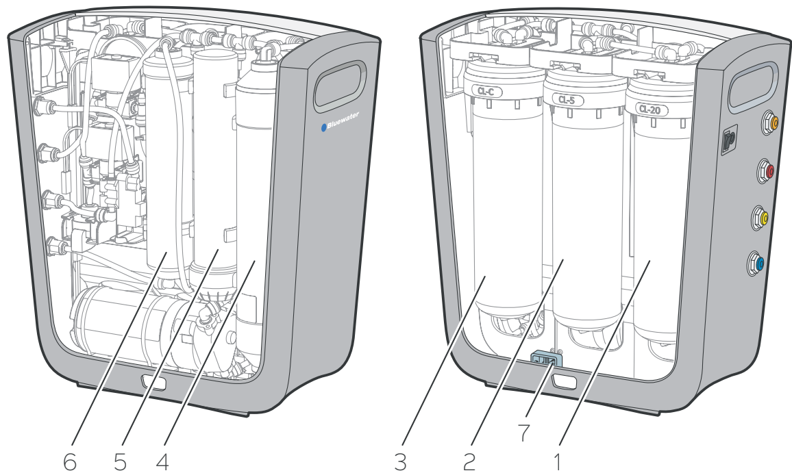
Bild 4. Cleones insida
