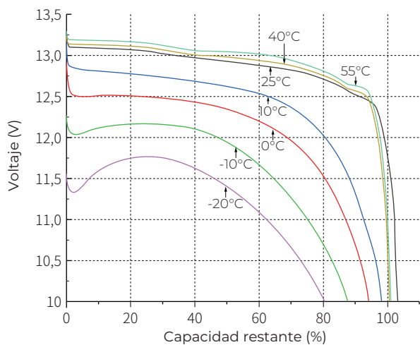
Capacidad de descarga a 0,5C a diferentes temperaturas
