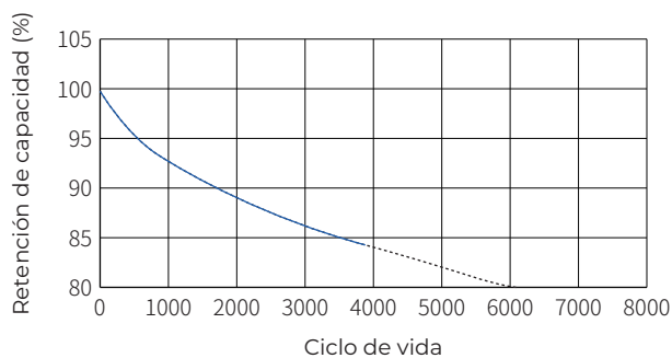
Ciclos de vida a 0,5C, 77 °F (25 °C)
