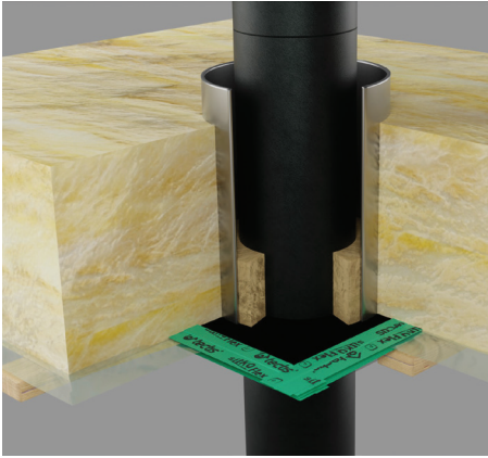
Periaatekuva metallisavupiipun yläpohjan läpiviennistä; HärmäAir.
