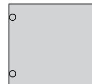
11 ( 15 x 495 x 491 mm) - 2x
