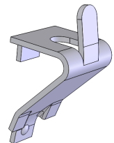
SHELF CLIP 290-0191
