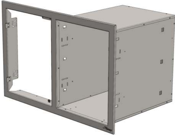
BODY 510-1173
