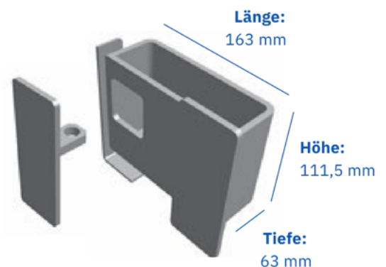
Materialstärke: 6 mm
