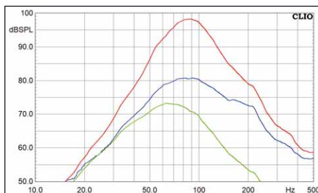
Der Bassboost ist mit 80 Hz zu hoch eingestellt, um effektiv Tiefgang zu bringen. Für das kleine Gehäuse erzielt der US 08 Active eine bemerkenswerte Grenzfrequenz
