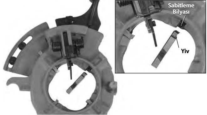
Şekil 16 – Paftaların Takılması
