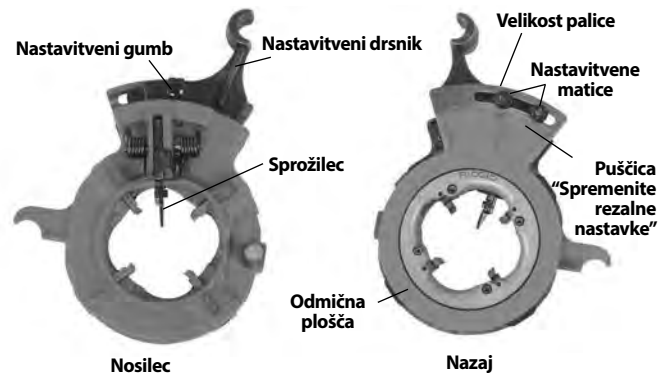
Slika 15 – Odtegotanje navojnih rezalnikov s samodejnim odpiranjem
