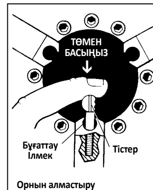
31-сурет – Қысқыш ендірмелерді ауыстыру
