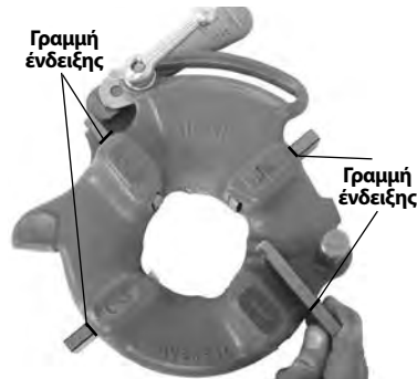
Εικόνα 8 – Τοποθέτηση μαχαιριών
