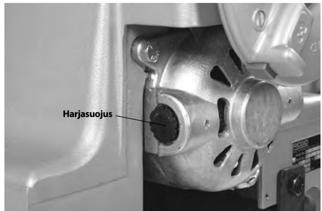
Kuva 32 – Moottorin kannen irrotus/Harjojen vaihto
