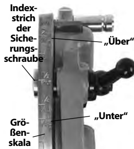
Abbildung 13 – Einstellen der Gewindegöße
