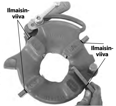
Kuva 8 – Terien asentaminen
