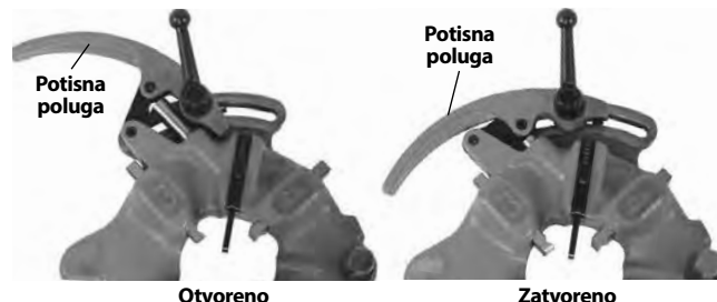
Slika 11 – Otvorena/zatvorena pozicija
