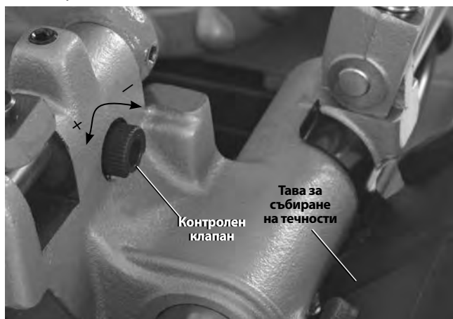
Фигура 5 – Регулиране на масления поток
