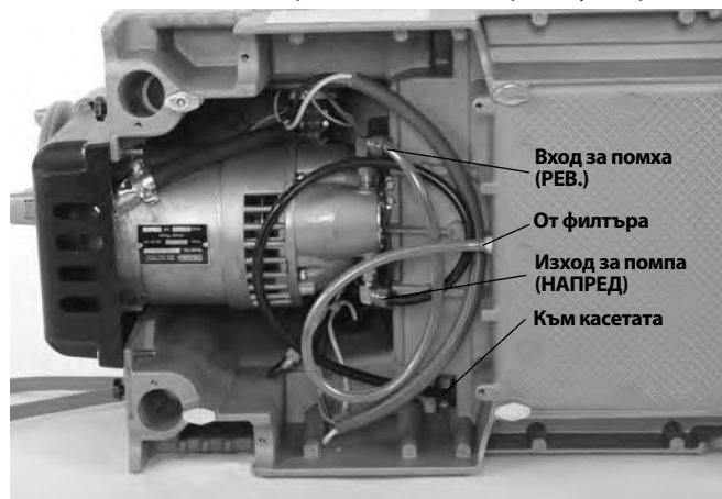
Фигура 25А – Връзка на маслената помпа за лява резба (Превключвател в позиция REV)
