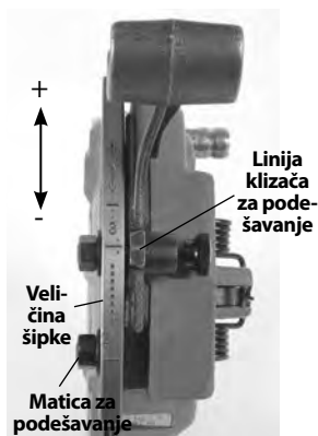
Slika 17 – Podešavanje veličine nareza
