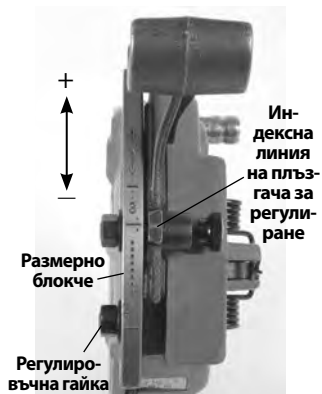
Фигура 17 – Регулиране на размера на резбата
