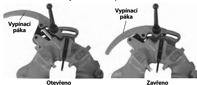
Obrázek 11 – Otevřená/zavřená poloha
