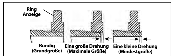
Abbildung 27 – Überprüfen der Gewindegröße
