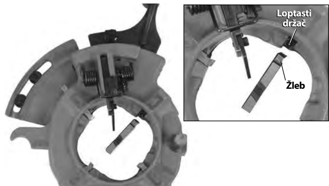
Slika 16 – Postavljanje noževa
