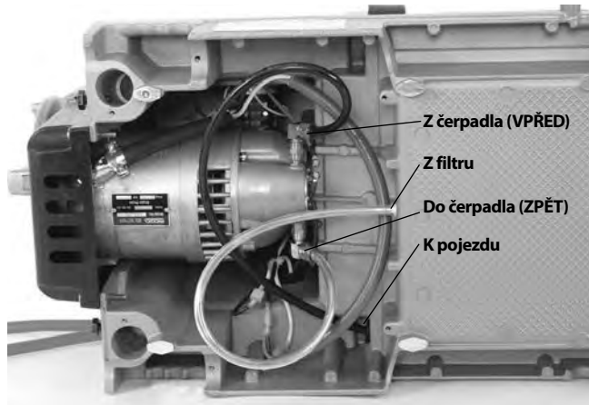
Obrázek 25B – Zapojení olejového čerpadla pro řezání pravotočivých závitů (spínač v poloze VPŘED)
