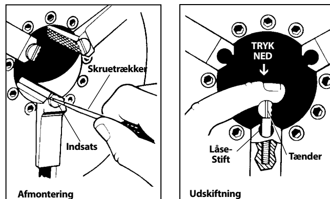
Figur 31 – Udskiftning af kæbeindsatse
