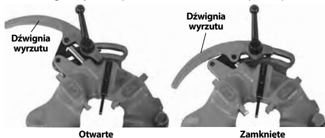
Rys. 11 – Położenie otwarcie/zamknięcie
