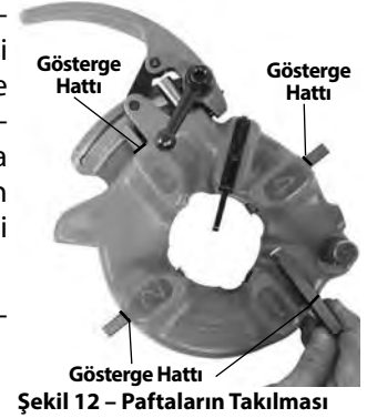
Şekil 12 – Paftaların Takılması
