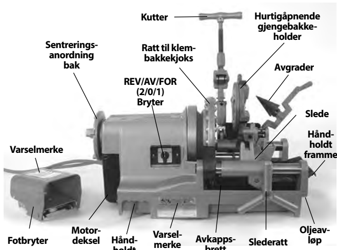
Figur 1 – 300 Compact gjengemaskin
