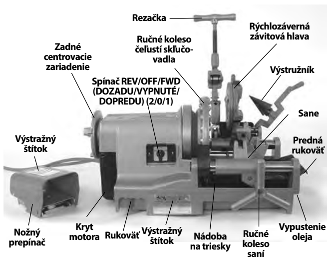
Obrázok 1 – Závítorez 300 Compact
