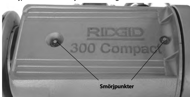
Figur 29 – Smörjpunkter
