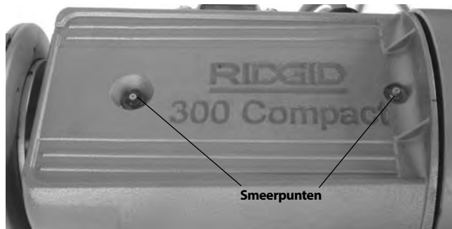
Afbeelding 29 – Smeerpunten
