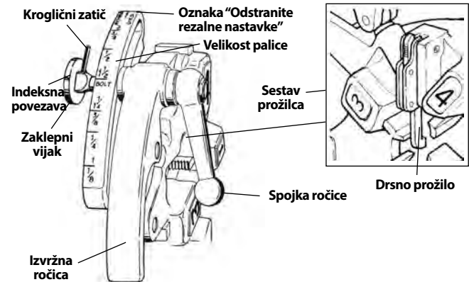
Slika 10 – Univerzalni samo-odpirajoč navojni rezalnik
