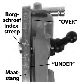
Afbeelding 13 – Schroefdraadmaatinstelling
