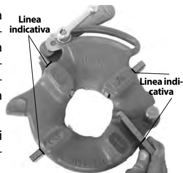
Figura 8 – Inserimento dei pettini
