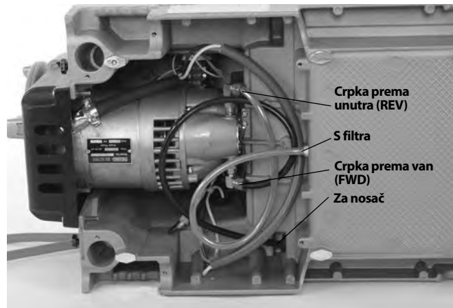
Slika 25A – Spojevi uljne crpke za narezivanje lijevih navoja (Prekidač u položaju REV)
