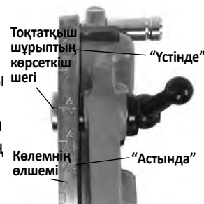
13-сурет – Бұранда өлшемін тексеру
