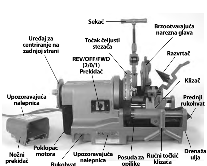
Slika 1 – 300 Compact mašinska nareznica
