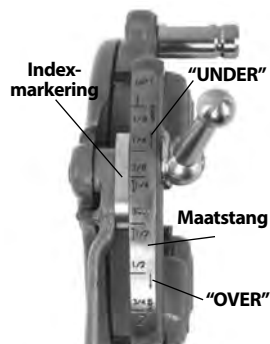
Afbeelding 9 – Schroefdraadmaat-instelling
