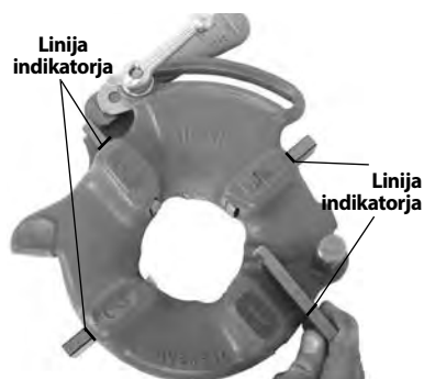
Slika 8 – Vstavljanje rezalnih nastavkov
