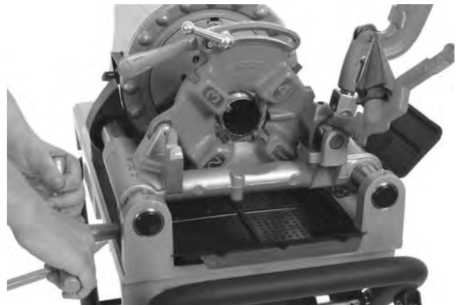
Фигура 24 – Резбоване на тръба (Показана е глава за матрици с бързо отваряне 811-A)
