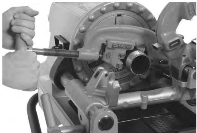
Фигура 22 – Рязане на тръба с нож
