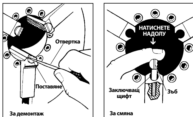
Фигура 31 – Смяна на вложките на челюстта
