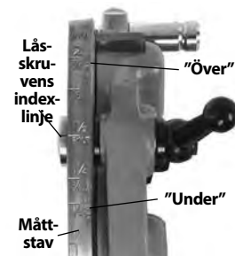
Figur 13 – Justera gängdimension
