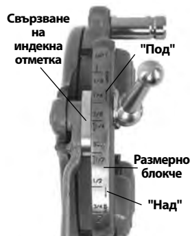
Фигура 9 – Регулиране на размера на резбата
