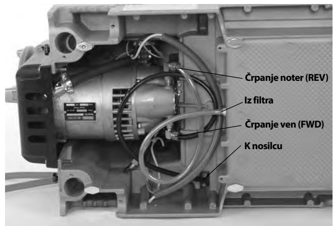
Slika 25A – Priključki črpalke za olje za levo-ročno rezanje navojev (Preklopite v REV)
