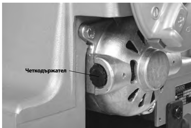
Фигура 32 – Отстраняване на капака на двигателя/ Смяна на четките
