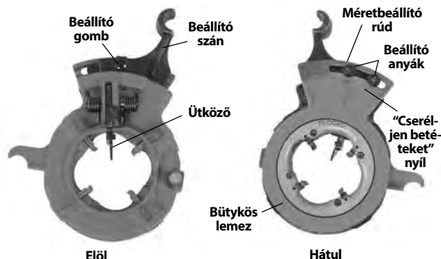
15. Ábra – Visszahúzódnőnyító menetvágófej
