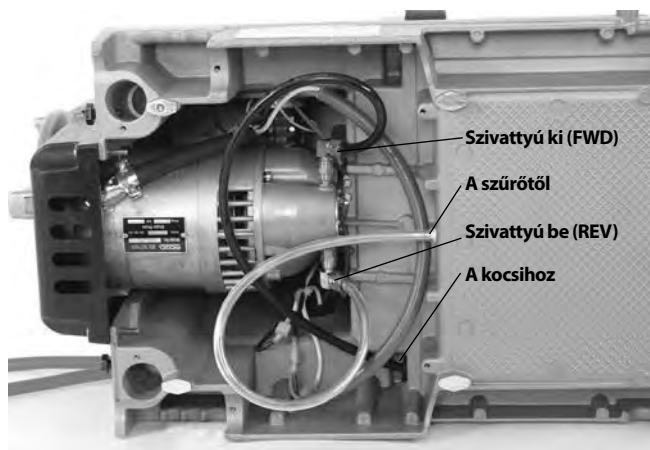
25B Ábra – Az olajszivattyú csatlakozásai jobbmenetűhöz (A kapcsoló FWD állásban)
