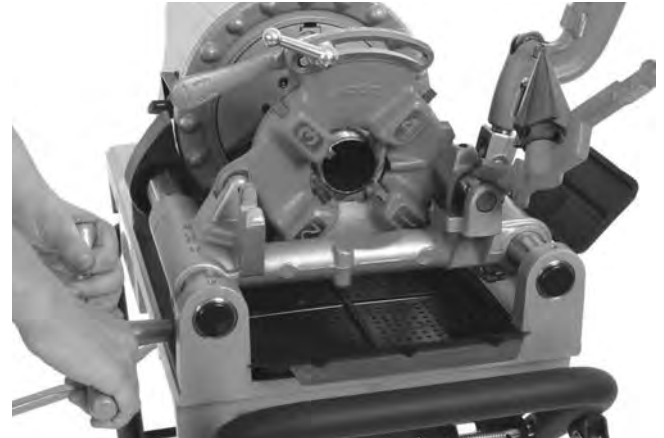
Figur 24 – Gevindskæring af rør (811-A hurtigt åbende skærehoved er vist)
