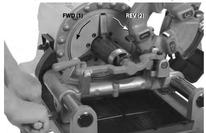
Slika 23 – Povrtanje cevi s povrtalnikom, rotacija naprave
