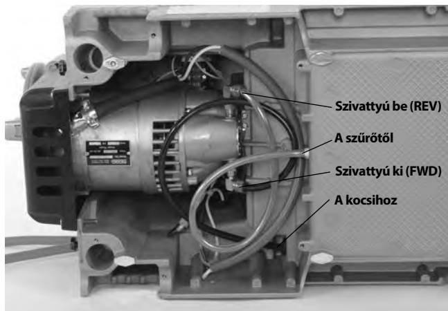
25A Ábra – Az olajszivattyú csatlakozásai balmenethez (A kapcsoló REV állásban)
