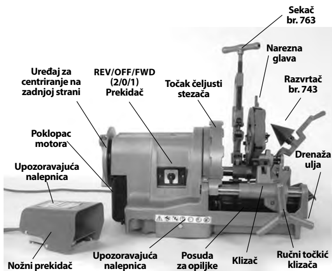
Slika 2 – 1233 mašinska nareznica
