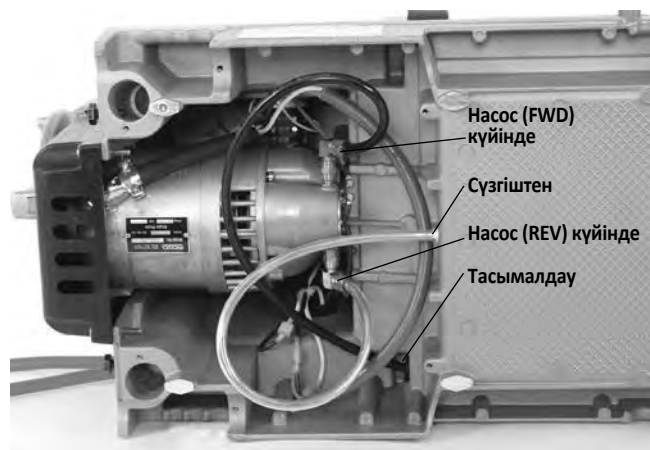
25B-сурет – Оң қолмен бұранда кесу үшін май сорғысының жалғамалары (қосқыш АЛҒА күйінде)
