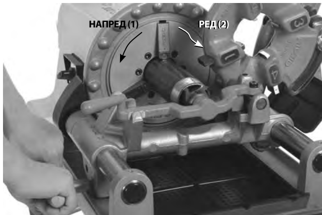
Фигура 23 – Разширяване на тръба с разширител, позиция на машината
