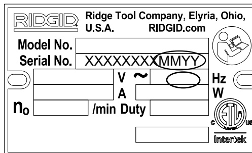
Сурет 3 – Құрылғының сериялық нөмірі
