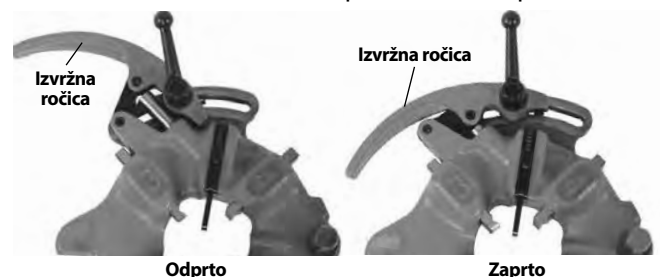
Slika 11 – Odprt/zaprt položaj
