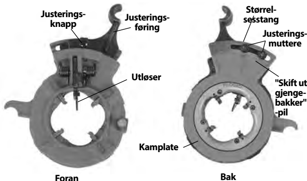
Figur 15 – Skrånende selvåpnende gjengebakkeholder
