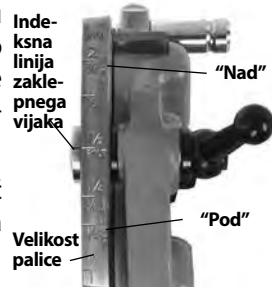
Slika 13 – Nastavljanje velikosti navoja
