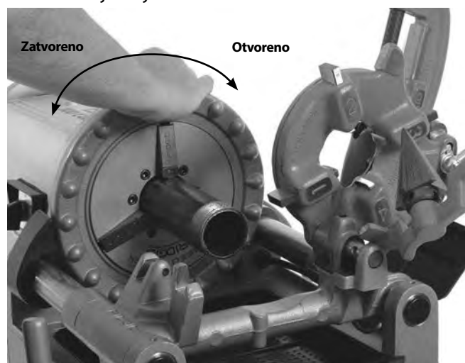
Slika 20 – Narezivanje cevi
