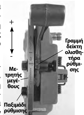
Εικόνα 17 – Ρύθμιση μεγέθους σπειρώματος
