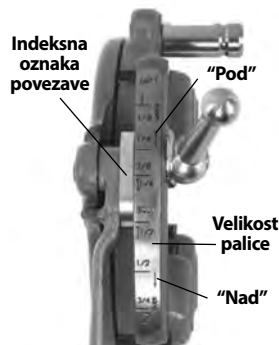
Slika 9 – Nastavljanje velikosti navoja
