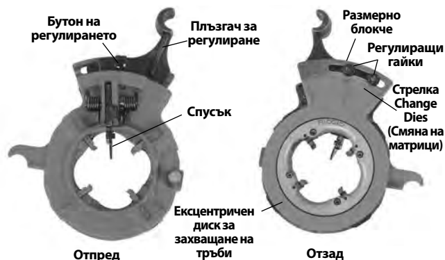
Фигура 15 – Падаща глава за матрици със самостоятелно отваряне
