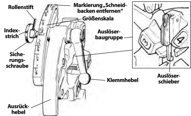
Abbildung 10 – Selbstöffnender Universalschneidkopf
