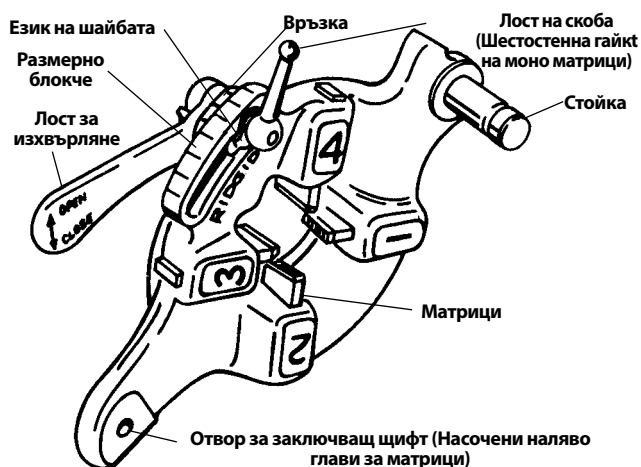
Фигура 6 – Глава за матрици с бързо отваряне
