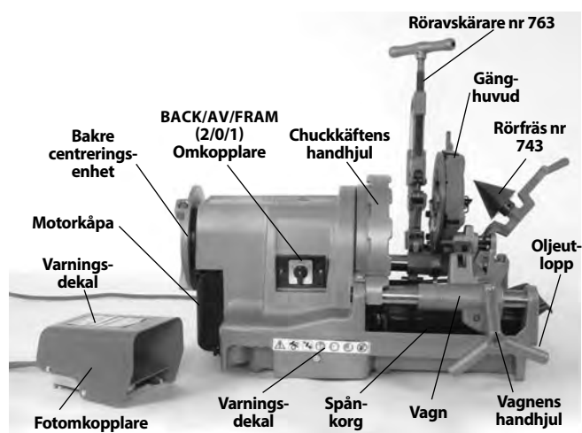
Figur 2 – 1233 gängmaskin
