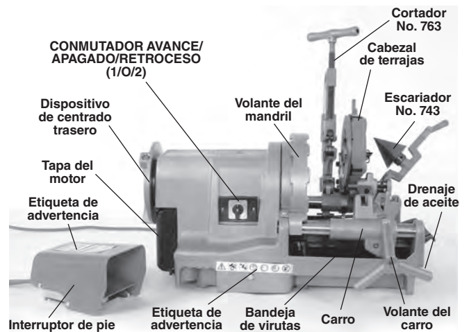
Figura 2 – Roscadora 1233
