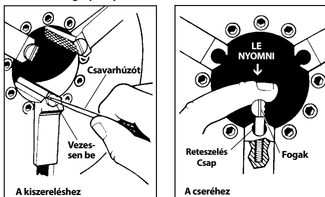
31. Ábra – Pofabetétek cseréje
