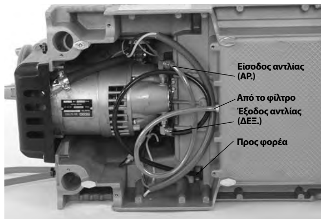
Εικόνα 25Α – Συνδέσεις αντλίας λαδιού για ελικοτόμηση αριστερού σπειρώματος (διακόπτης στο ΑΡ.)
