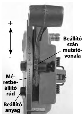
17. Ábra – A menet méretének beállítása
