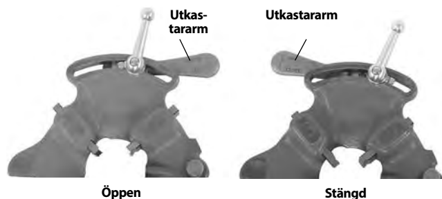
Figur 7 – Öppen/stängd armposition
