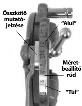
9. Ábra – A menet méretének beállítása
