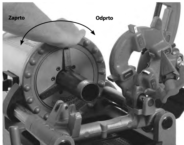
Slika 20 – Cev glave
