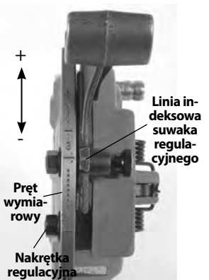
Rys. 17 – Regulacja wymiaru gwintu
