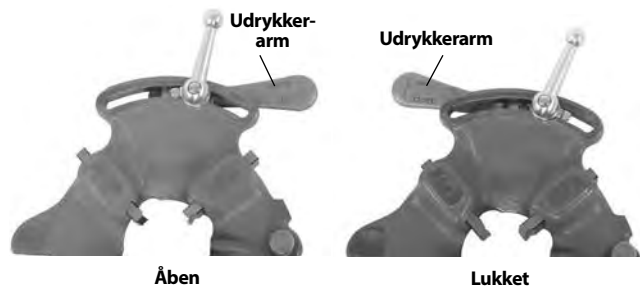
Figur 7 – Åben/lukket armstilling
