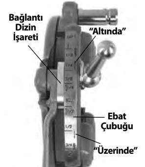
Şekil 9 – Diş Boyutunun Ayarlanması
