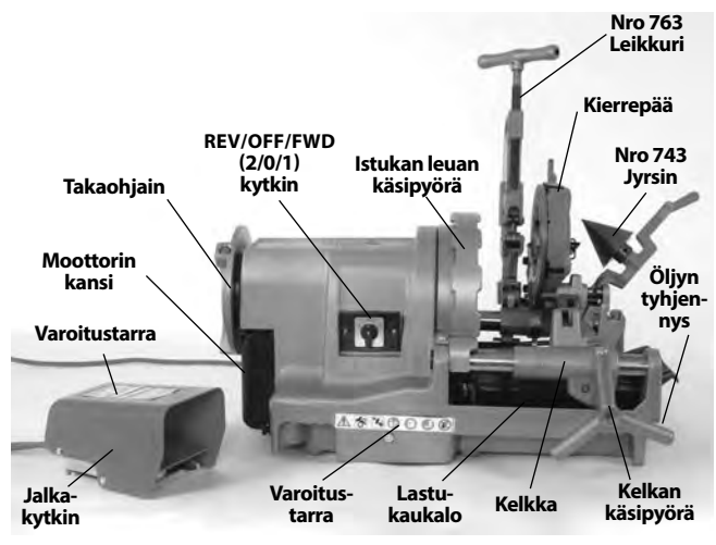
Kuva 2 – 1233-kierteityskone
