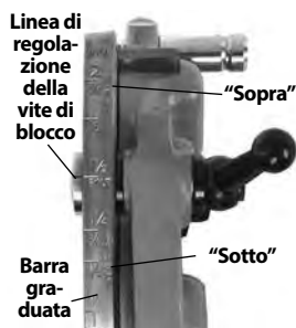
Figura 13 - Regolazione della dimensione della filettatura
