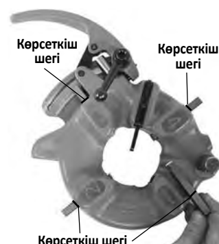
12-сурет – Бастиектерді енгізу
