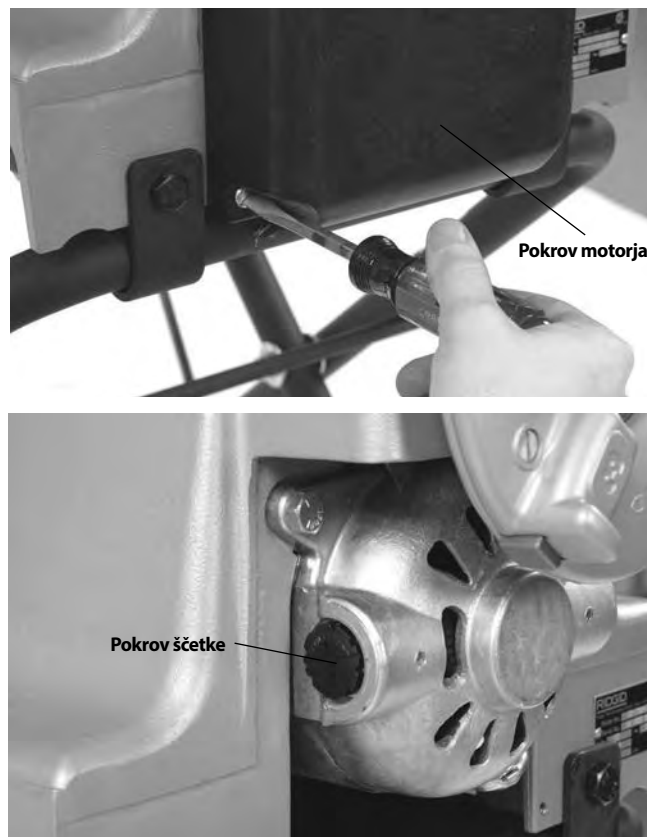
Slika 32 – Odstranjevanje pokrova motorja/zamenjava ščetk
