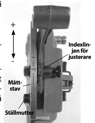
Figur 17 – Justera gängdimension
