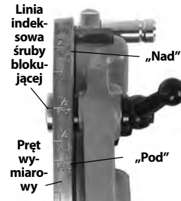
Rys. 13 – Regulacja wymiaru gwintu
