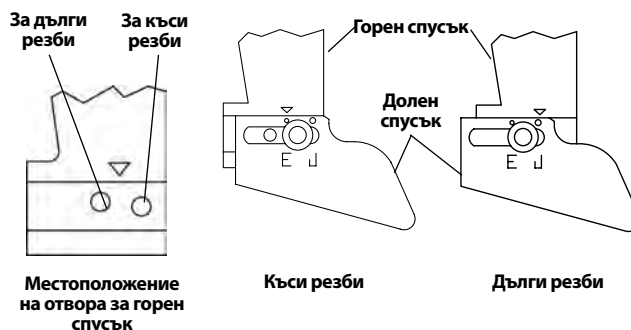
Фигура 18 – Регулиране на дължината на резбата
