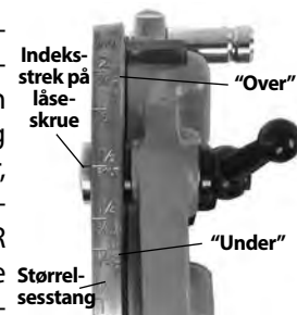
Figur 13 - Justering av gjengestørrelse
