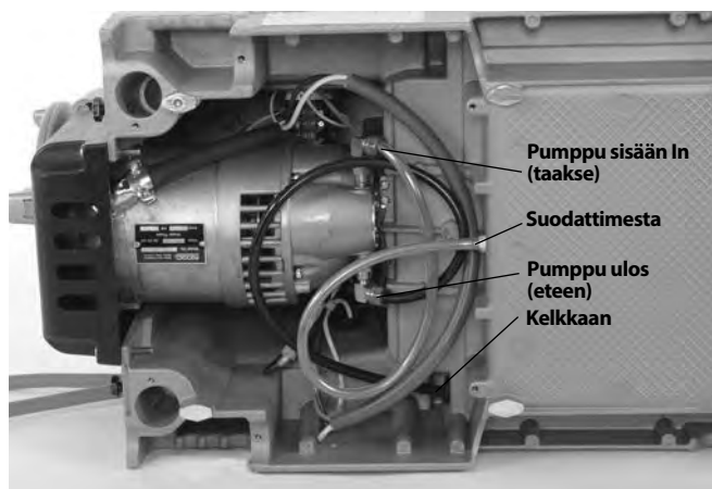
Kuva 25A – Öljypumpun liitännät vasenkätiseen kierteykseen (kytkin asennossa REV (taakse))
