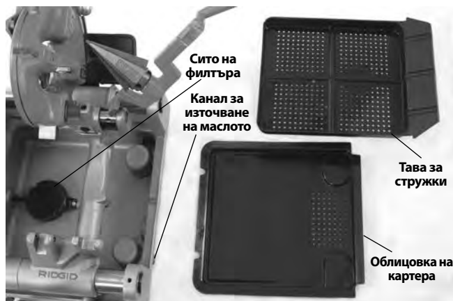
Фигура 30 – Сглобка на ситото на филтъра
