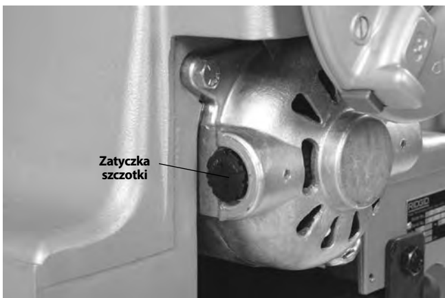
Rys. 32 – Zdejmowanie pokrywy silnika/Zmiana szczotek
