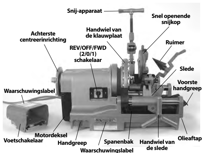
Afbeelding 1 – 300 Compact schroefdraadsnijmachine
