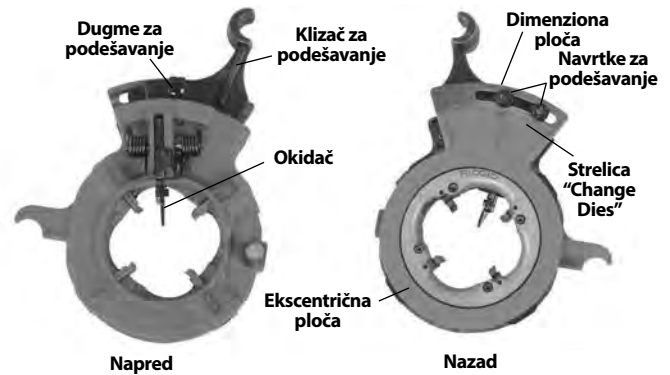
Slika 15 – Samootvarajuća narezna glava sa uzmicanjem noževa
