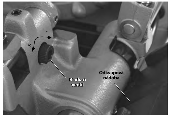
Obrázok 5 – Nastavenie toku oleja
