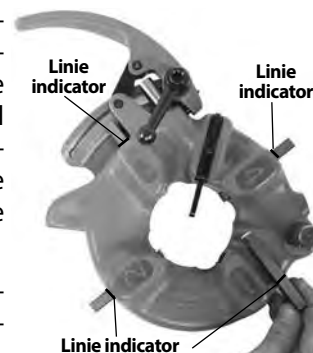
Figura 12 – Inserare filiere
