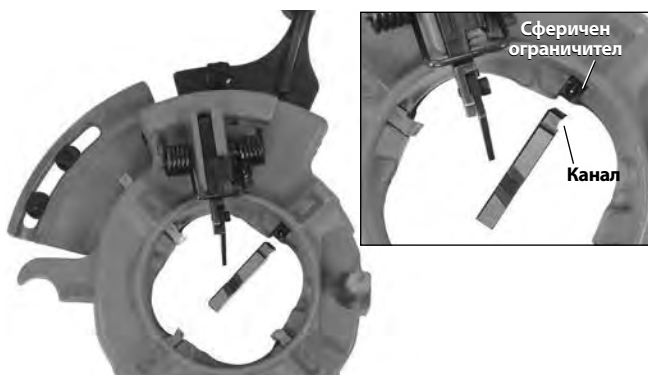
Фигура 16 – Поставяне на матрици
