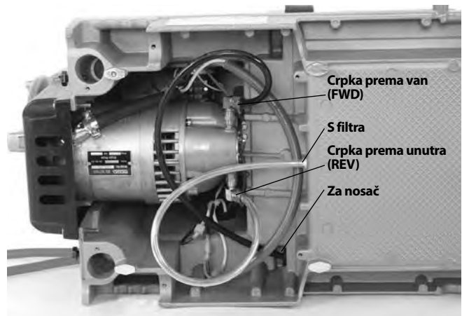
Slika 25B – Spojevi uljne crpke za narezivanje desnih navoja (Prekidač u položaju FWD)
