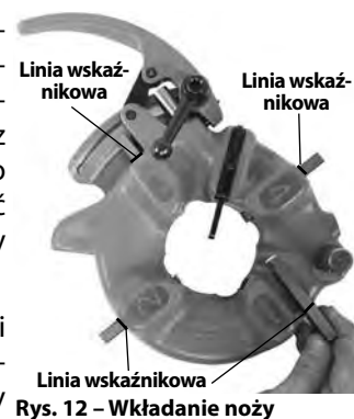
Rys. 12 – Wkładanie noży
