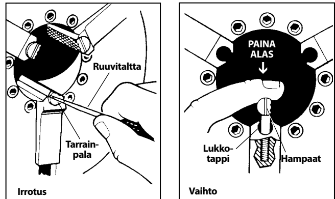
Kuva 31 – Leuan tarrainpalojen vaihtaminen
