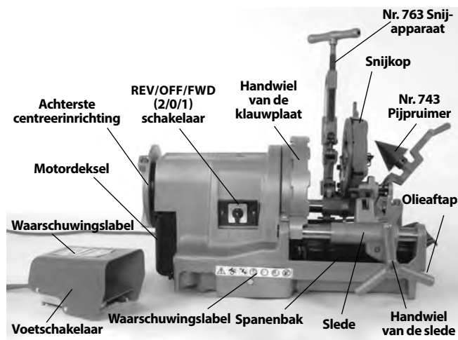
Afbeelding 2 – 1233 schroefdraadsnijmachine
