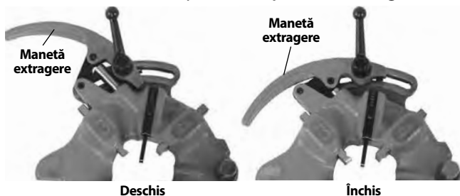
Figura 11 – Pozițiile Deschis/Închis
