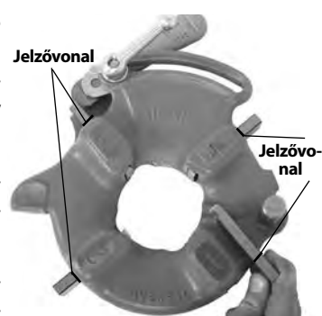
8. Ábra – Betétek behelyezése
