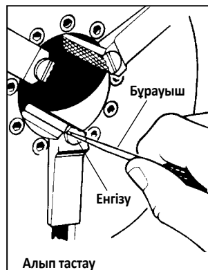
31-сурет – Қысқыш ендірмелерді ауыстыру
