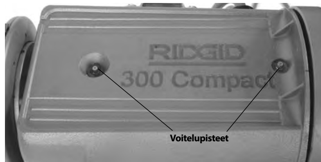
Kuva 29 – Voitelupisteet
