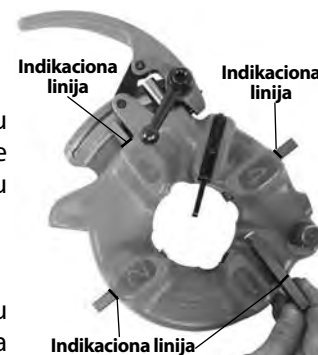
Slika 12 – Postavljanje noževa
