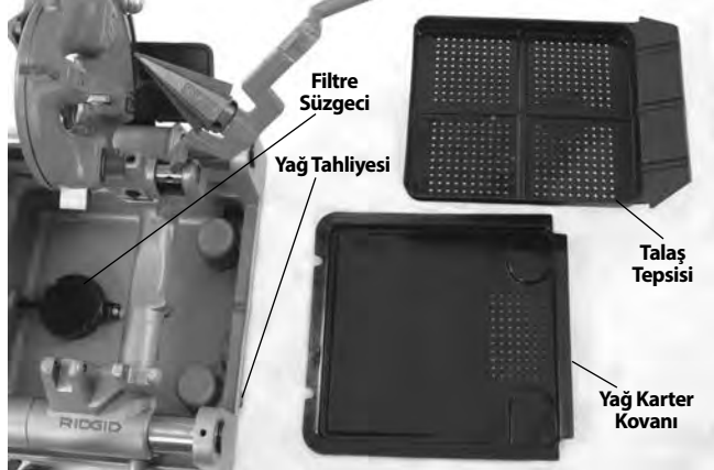
Şekil 30 – Filtre Süzgeç Düzenliği
