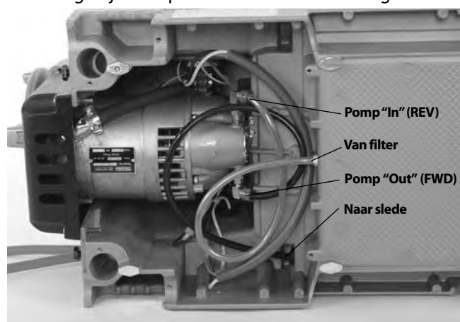
Afbeelding 25A – Oliepompaansluitingen voor het snijden van linkse schroefdraad (schakelaarstand REV)
