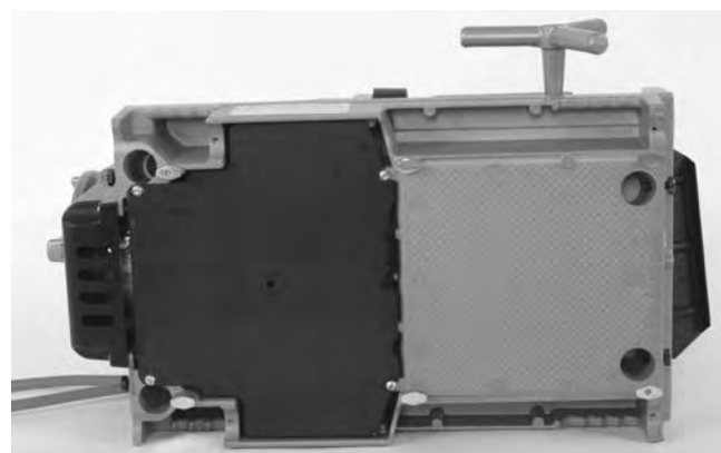
Figur 25C – Skydd på plats
