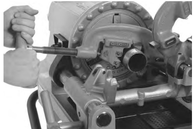
Slika 22 – Rezanje cevi z rezilom
