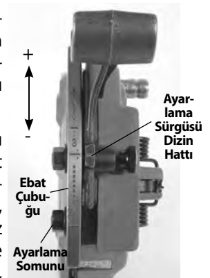
Şekil 17 – Diş Boyutunun Ayarlanması
