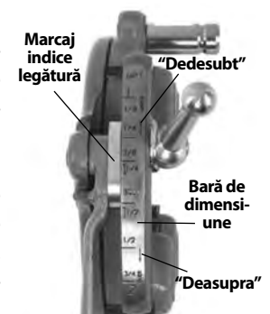
Figura 9 – Verificare dimensiune filet
