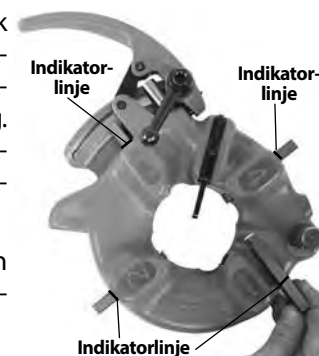
Figur 12 – Sette inn gjengebakker
