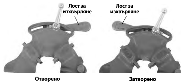
Фигура 7 – Позиция на лоста за отваряне/затваряне
