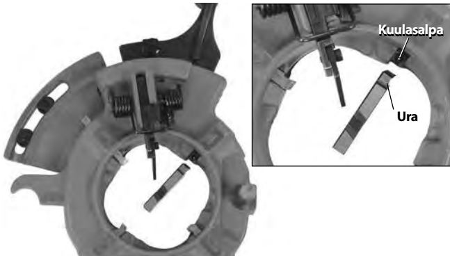
Kuva 16 – Terien asentaminen
