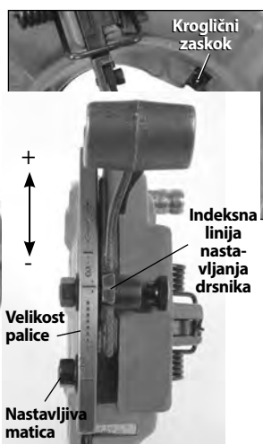
Slika 17 – Nastavljanje velikosti navoja
