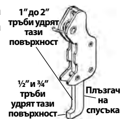
Фигура 14 – Настройка на спусъка
