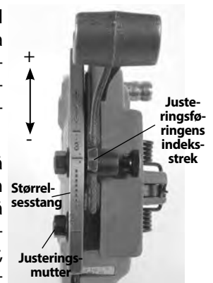
Figur 17 – Justering av gjengestørrelse
