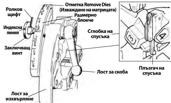
Фигура 10 – Универсална самоотваряща се глава за матрици
