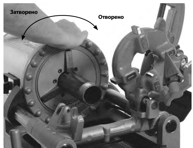
Фигура 20 – Захващане на тръба в патронника
