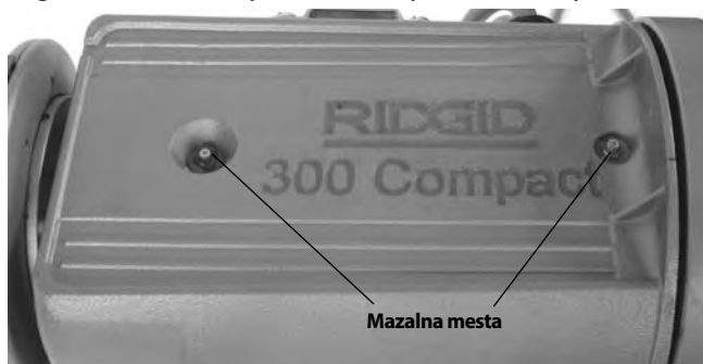
Slika 29 – Mazalna mesta
