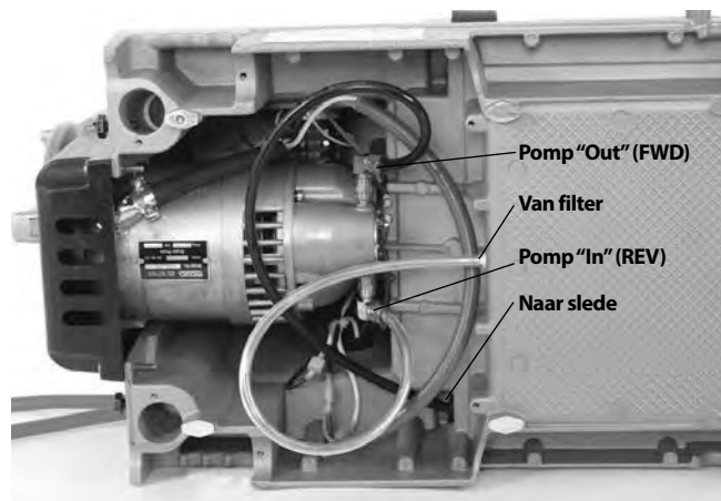
Afbeelding 25B – Oliepompaansluitingen voor het snijden van rechtse schroefdraad (schakelaarstand FWD)
