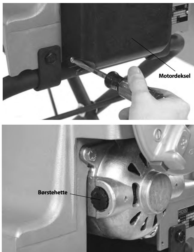
Figur 32 – Fjerne motordeksel/skifte ut børster
