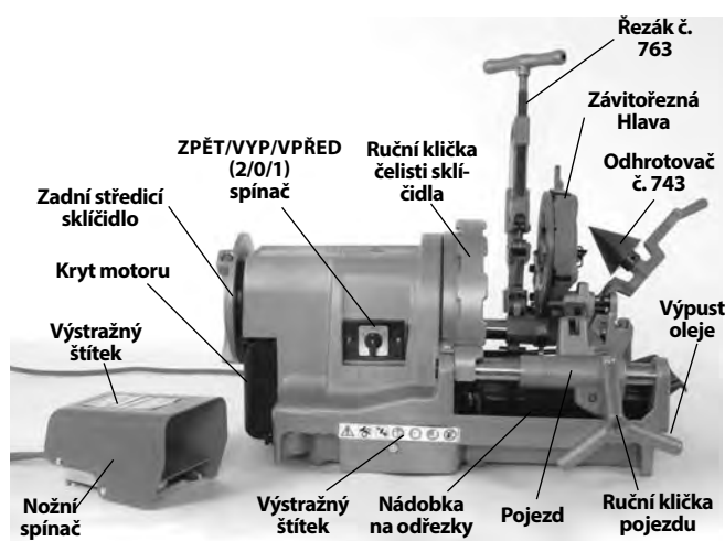
Obrázek 2 – Závitorezný nástroj 1233
