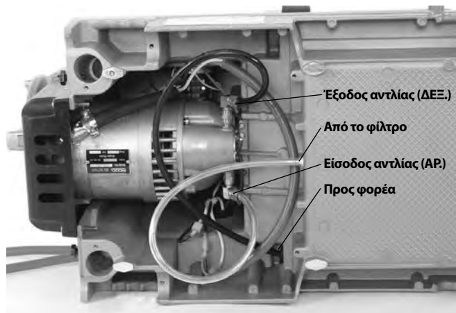
Εικόνα 25Β – Συνδέσεις αντλίας λαδιού για ελικοτόμηση δεξιού σπειρώματος (διακόπτης στο ΔΕΞ.)
