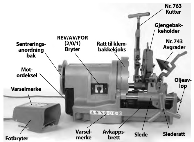
Figur 2 – 1233 Gjengemaskin
