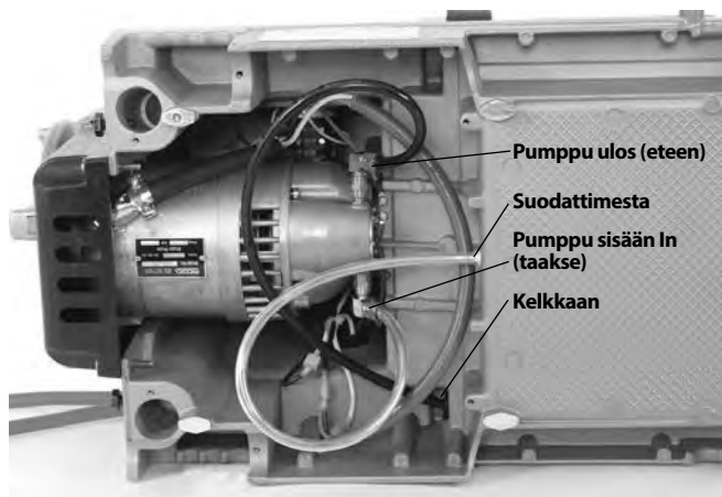
Kuva 25B – Öljypumpun liitännät oikeakätiseen kierteykseen (kytkin asennossa FWD (eteen))
