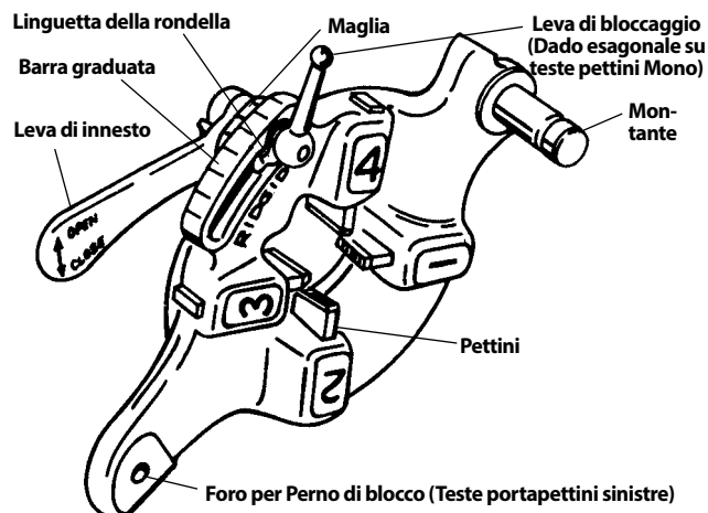
Figura 6 – Testa portapettini ad apertura rapida
