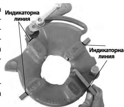
Фигура 8 – Поставяне на матрици
