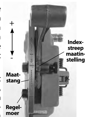
Afbbeelding 17 – Schroefdraadmaatinstelling
