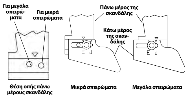
Εικόνα 18 – Ρύθμιση μεγέθους σπειρώματος
