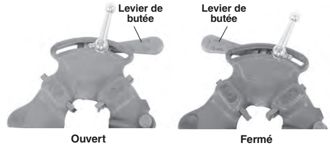
Figure 7 – Levier ouvert/fermé
