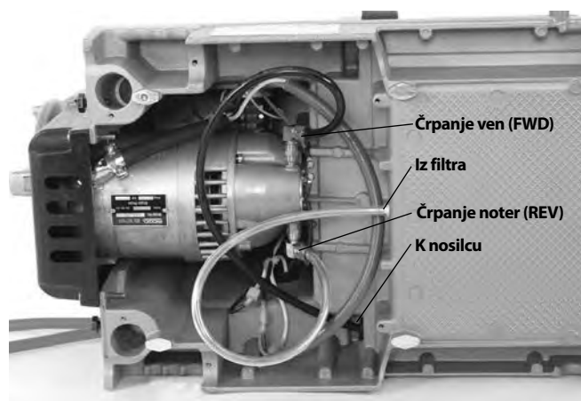
Slika 25B – Priklučki črpalke za olje za desno-ročno rezanje navojev (Preklopite v FWD)
