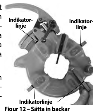
Figur 12 – Sätta in backar
