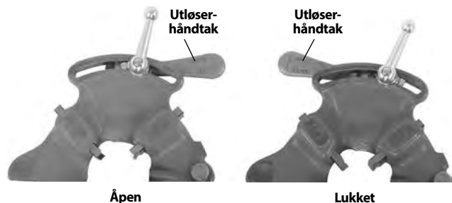
Figur 7 – Åpen/lukket-håndtaksposisjon
