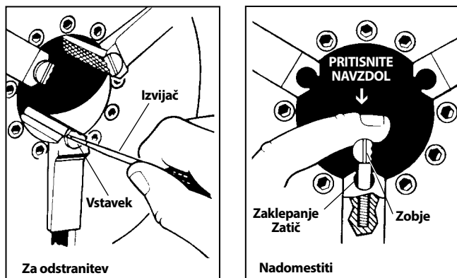
Slika 31 – Zamenjava rezalnih vstavkov
