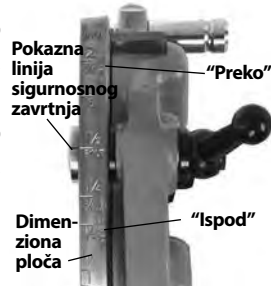
Slika 13 – Podešavanje veličine navoja
