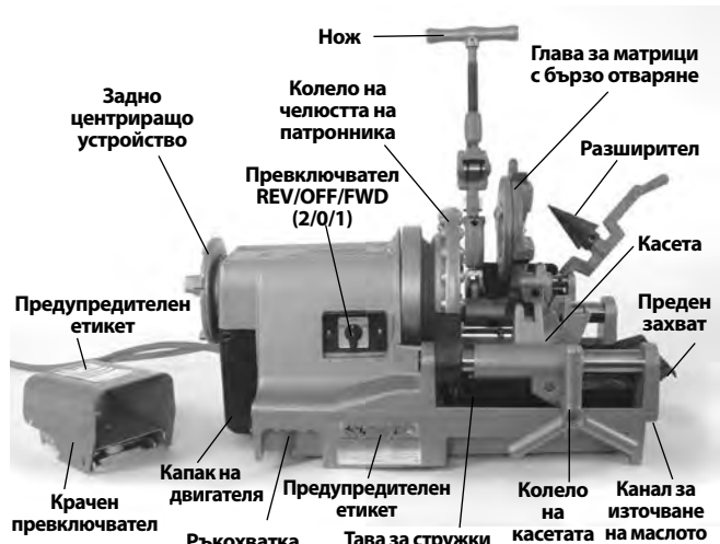
Фигура 1 – Винтонарезни машини 300 Compact
