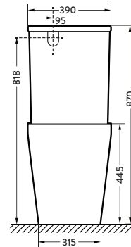
S-TRAP 80mm-245mm
