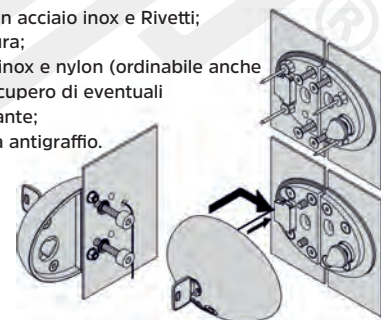
Esempio installazione dell'antifurto F638665 (A) senza gruppo di fissaggio F638662 .
