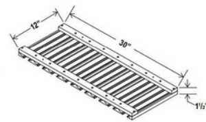
SGH30
