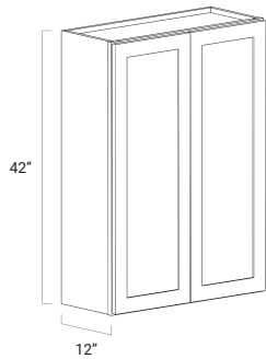
W2442/W2742/W3042/ W3342/W3642/W3942
