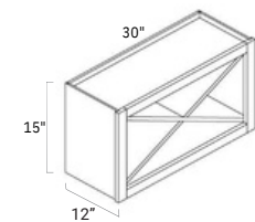
WRC3015
