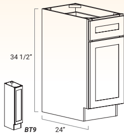
BT9/B12/B15/B18/B21
