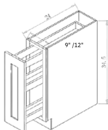
BSPR9/BSPR12
