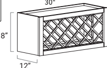
WRC3018/WRC2430
