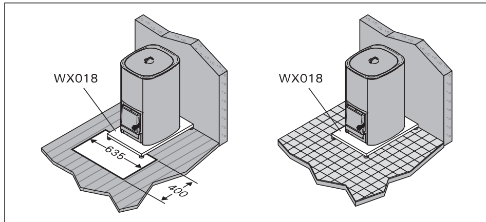
Figure 4. Protecting the floor (all dimensions in millimeters) Рисунок 4. Защита пола (все размеры приведены в миллиметрах)
