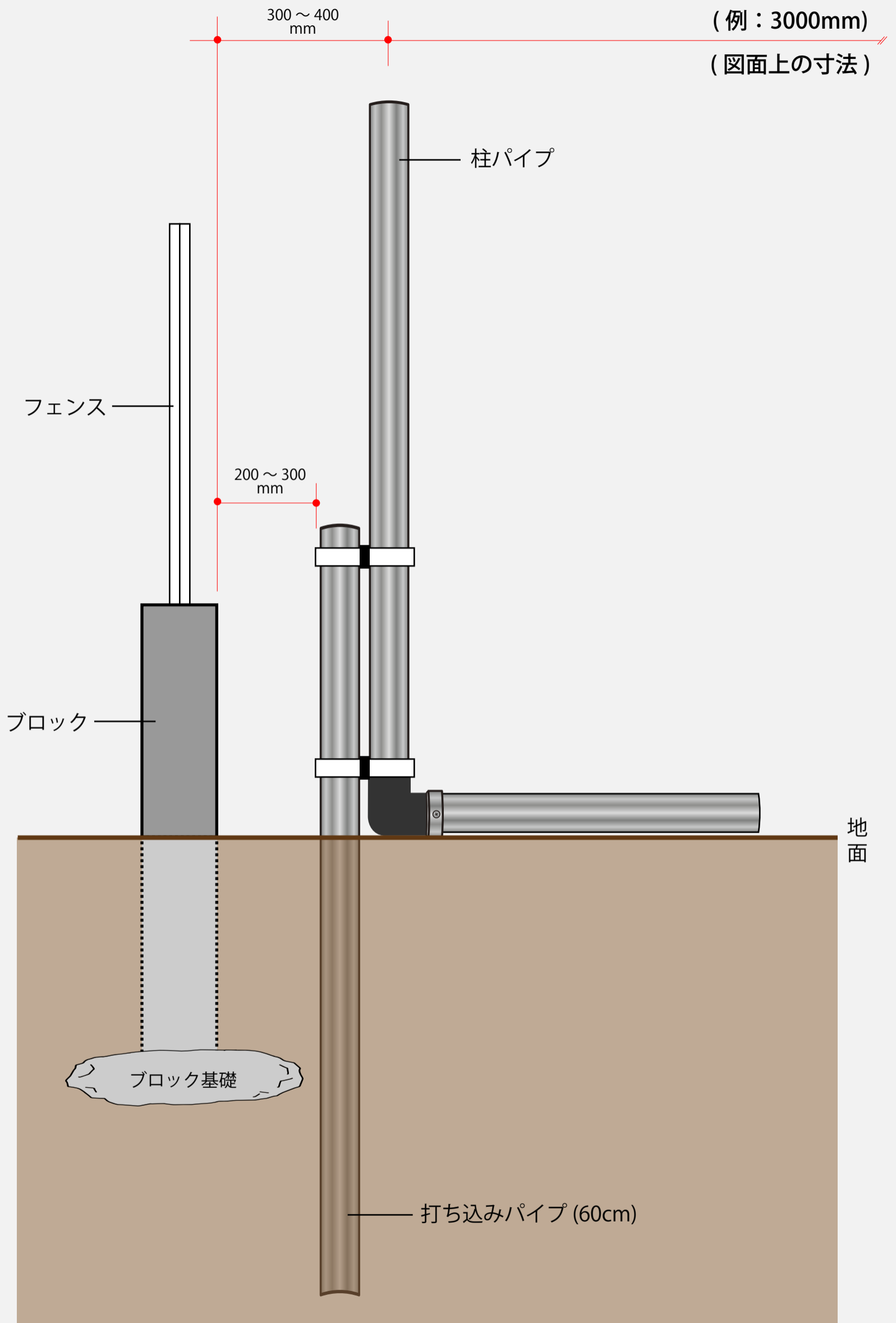
[ 立面図 ]
