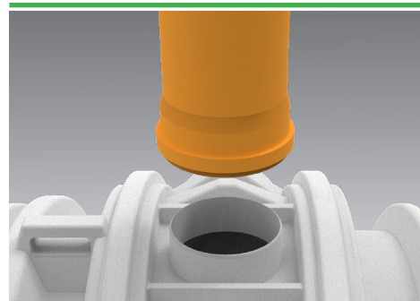
Ø250 rør med tilsluttet muffe
