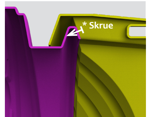
Overlap ved en lille ribbe og endemodul.
