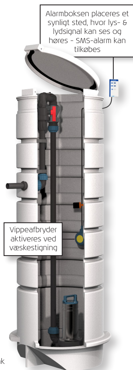
Eksempel på Ø600 spildevandsbrønd med VA-alarm
