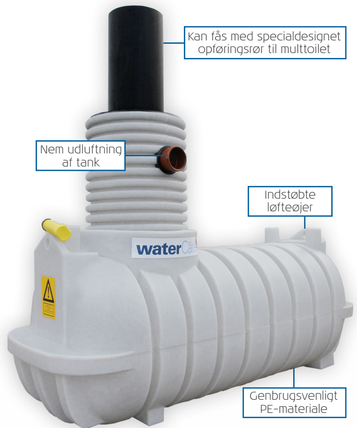
Eksempel på kundetilpasset WaterCare Samletank - 1.200 l. - Fås fra 600 til 7.000+ l
