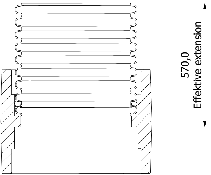
A-A ( 1 : 10 )
