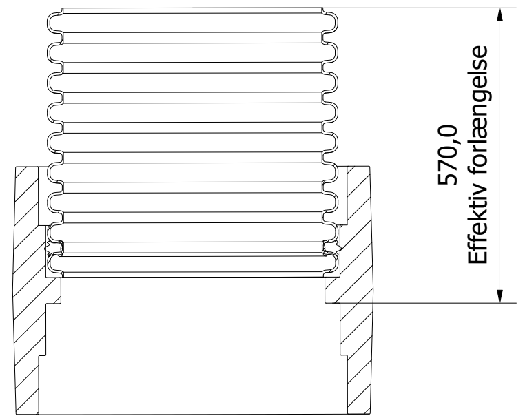
A-A ( 1 : 10 )
