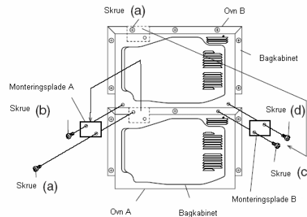
Fig. A: Sådan sammenkobles to ovne.
