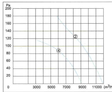
60Hz
