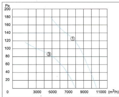
50Hz
